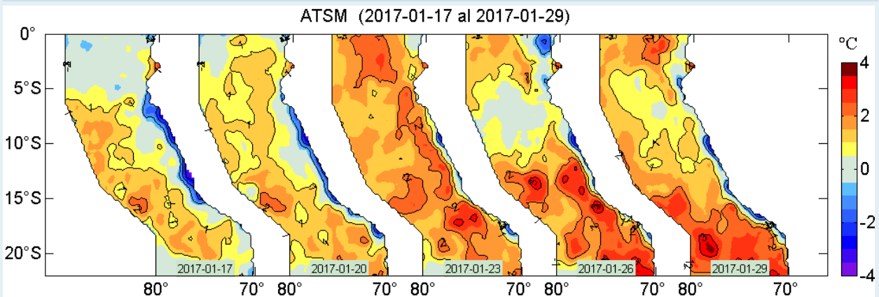
Figura 2. Anomalías de la temperatura superficial del agua (°C) en el mar peruano, cada tres días, entre el 17 y 29 de enero del 2017. Datos: AVHRR Global Reyn_SmithOiv2R (Reynolds, et. al., 2007) de CMB/EMC/NCEP de la NOAA. Procesamiento: IMARPE.
