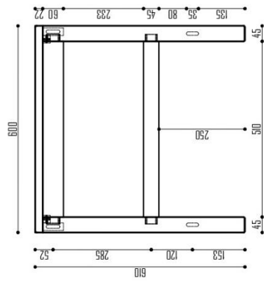
VISTA FRONTAL Escala 1 / 10
