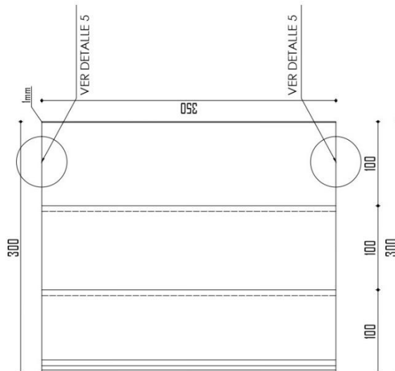
VISTA SUPERIOR
