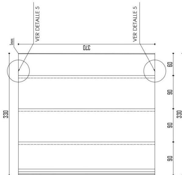
VISTA SUPERIOR Escala 1 / 4
