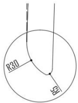
DETALLE 3 Escala 1 / 2
