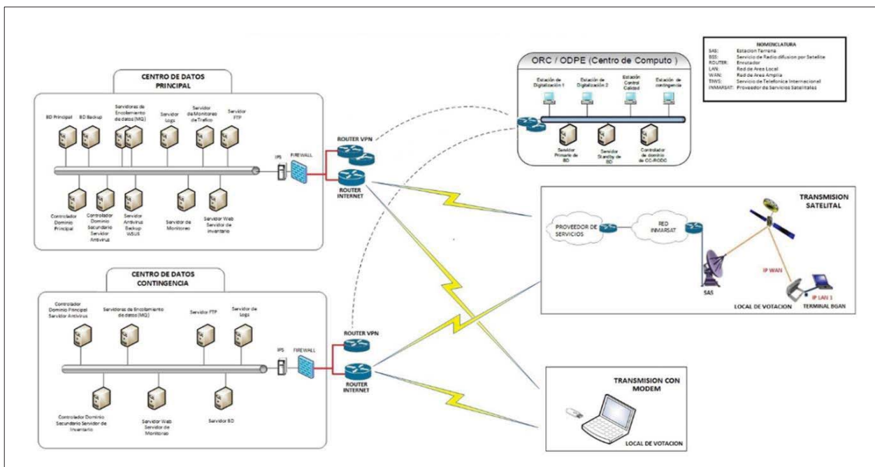
Figura N°7: Arquitectura de RED del SPAMD
