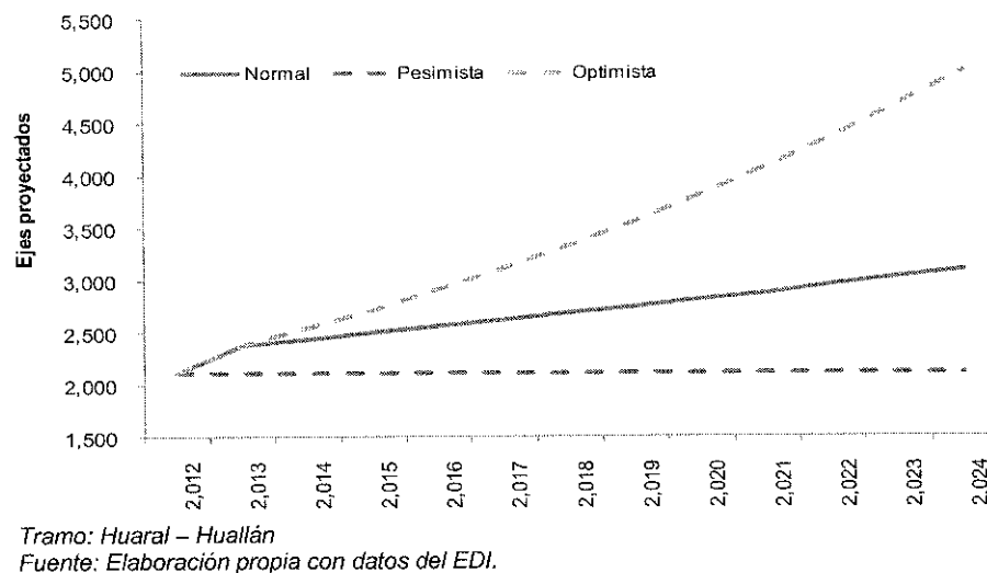
FIGURA 5: PROYECCIÓN DE TRÁFICO (EN EJES) POR TIPO DE VEHÍCULO (IMDA): TRAMO HUARAL – HUALLÁN
