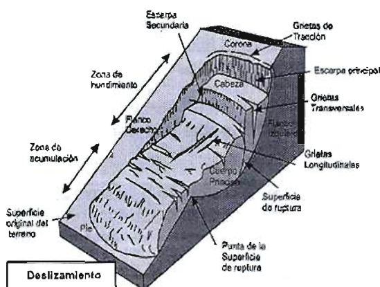
Figura N° 1 "Deslizamientos"
