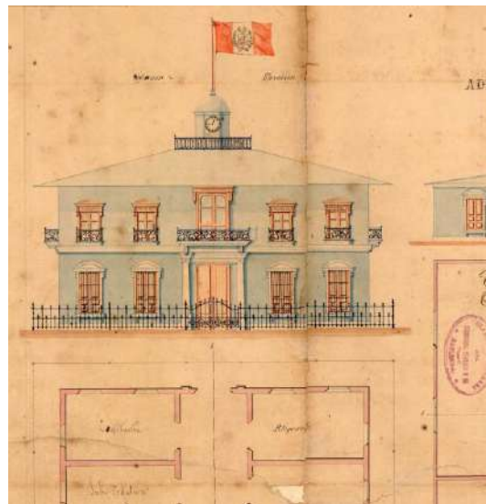
(57) PL046. Detalle de la Aduana de Paita
