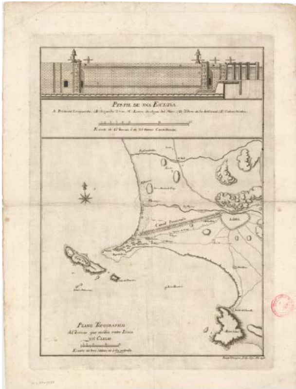
(6) PL10. Plano Topográfico entre Lima y el Callao.
