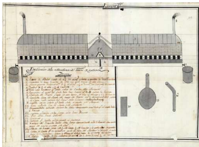
(32) PL102d. Máquina para extraer azogue
