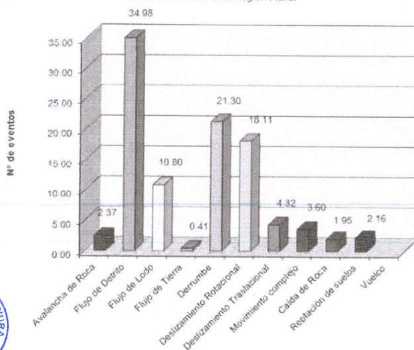
Gráfico 3 Distribución de movimientos en masa en la Región Piura.
