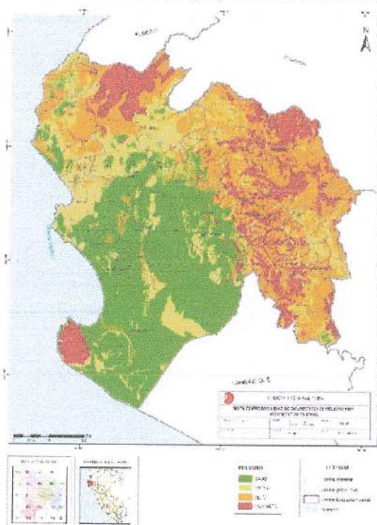
Mapa 6 Mapa de probabilidad de ocurrencia de peligro por movimientos en masa
