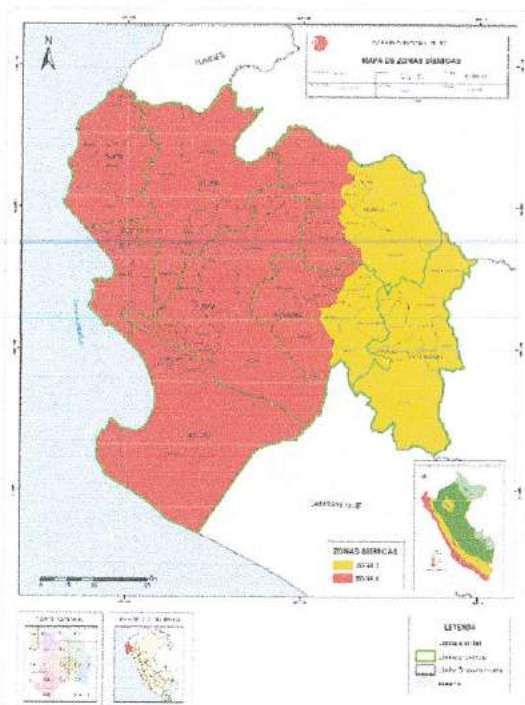
Mapa 7 Mapa de Zonas Sísmicas en la Región Piura
