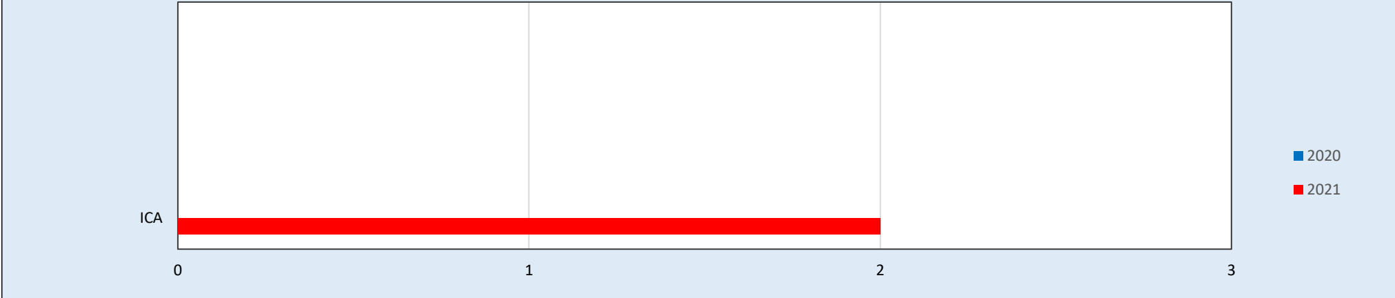
Gráfico N° 3. Distribución del número de brotes de ENC Semana epidemiológica 1 a 16. Comparativo Año 2020 - 2021
