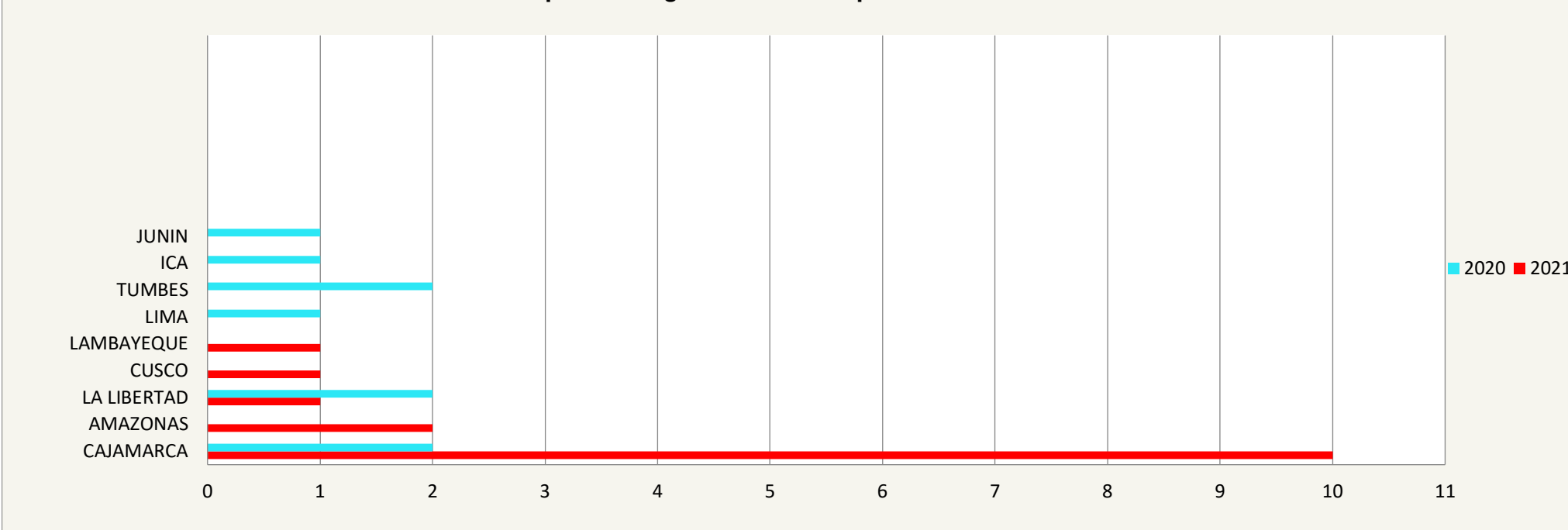
Gráfico N° 3. Distribución del número de brotes de ENC Semana epidemiológica 1 a 16. Comparativo Año 2020 - 2021
