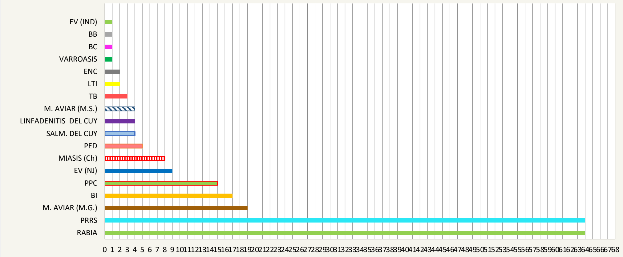
Gráfico N° 1. Número de brotes de enfermedades. (semana epidemiológica 16) Año 2021
