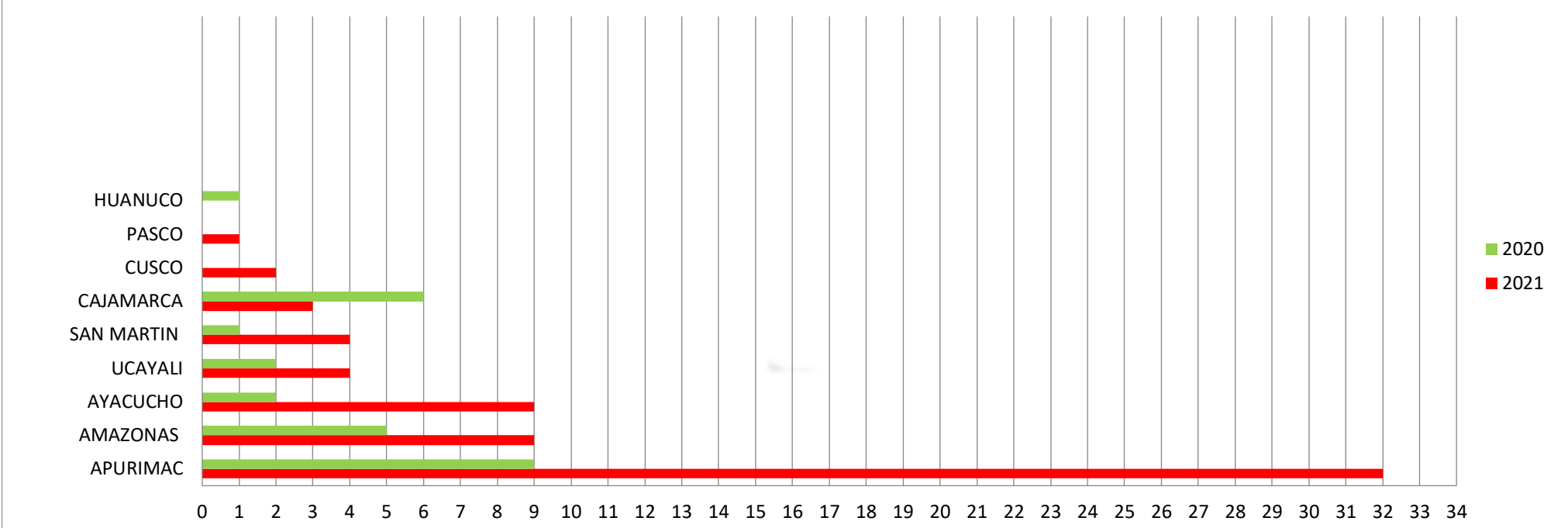
Gráfico N° 3. Distribución del número de brotes de PPC Semana epidemiológica 1 a 16. Comparativo Año 2020 - 2021
