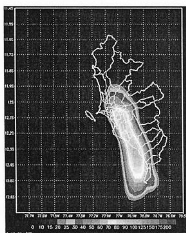
Grafico 3. Material Particulado de 10 \mu\text{m}^3 - PM 10 en Lima Sur
