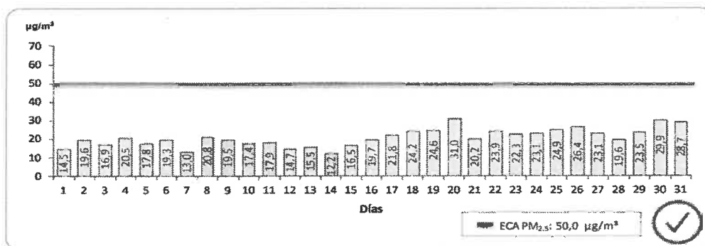
GRAFICO N° 16. LIMA ESTE. CONCENTRACION DIARIA DE MATERIAL PARTICULADO INFERIOR A 2,5 MICRAS, EN LA ESTACION DE MEDICIÓN DE CAMPO DE MARTE, MARZO 2021.
