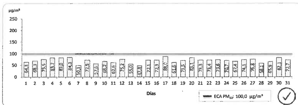
GRAFICO N° 15. LIMA ESTE. CONCENTRACION DIARIA DE MATERIAL PARTICULADO INFERIOR A 10 MICRAS, EN LA ESTACION DE MEDICIÓN DE CAMPO DE MARTE, MARZO 2021.
