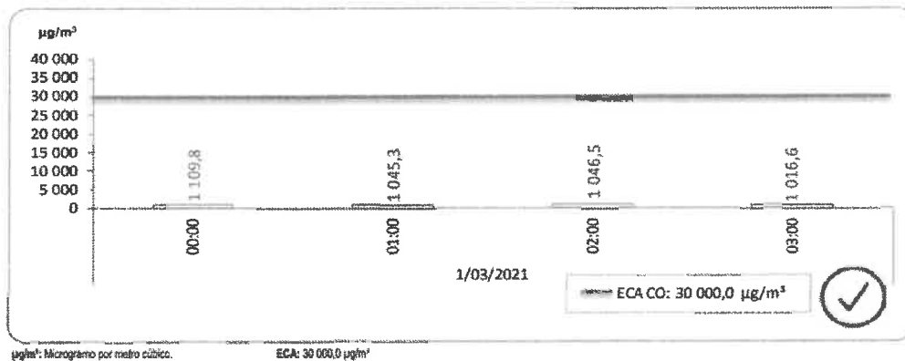
GRAFICO N° 17. LIMA ESTE. VALOR DE MONÓXIDO DE CARBONO (CO), EN LA ESTACION DE MEDICIÓN DE SAN JUAN DE LURIGANCHO, MARZO 2021.
