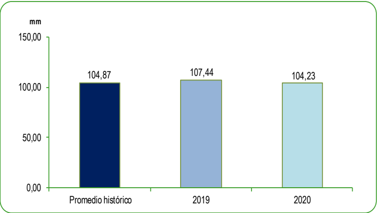
GRÁFICO N°35 PERÚ: PROMEDIO DE LAS PRECIPITACIONES EN LA VERTIENTE DEL LAGO TITICACA Mes: Diciembre 2019 - 2020 Milímetros (mm)
