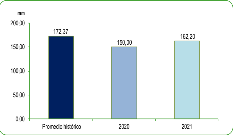
GRÁFICO N°43 PERÚ: PROMEDIO DE LAS PRECIPITACIONES EN LA VERTIENTE DEL LAGO TITICACA Mes: Enero 2020 - 2021 Milímetros (mm)
