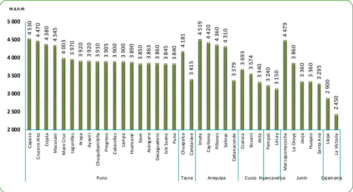
GRÁFICO N°43 PERÚ: ALTITUD DE LAS ESTACIONES METEOROLÓGICAS Metros sobre el nivel del mar
