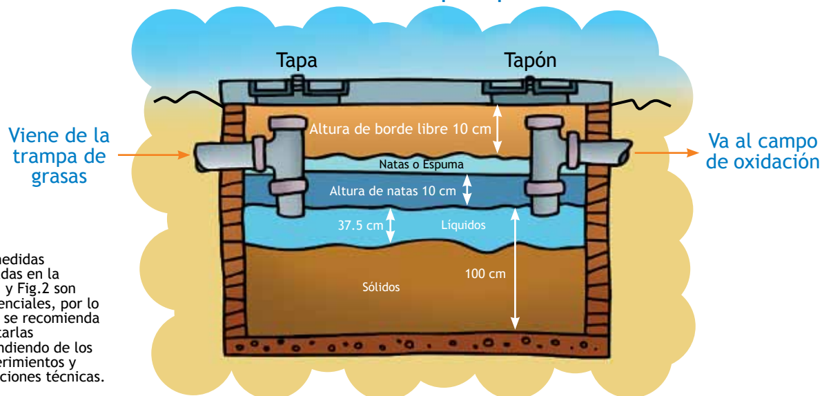
FIGURA N° 2. Tanque séptico
