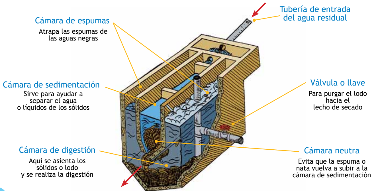
FIGURA N° 3. Tanque Imhoff
