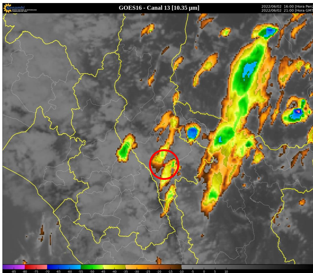
Figura 1: Imagen de Satélite GOES16 en el Canal infrarrojo del 02 de junio de 2022 –16:00 horas.
