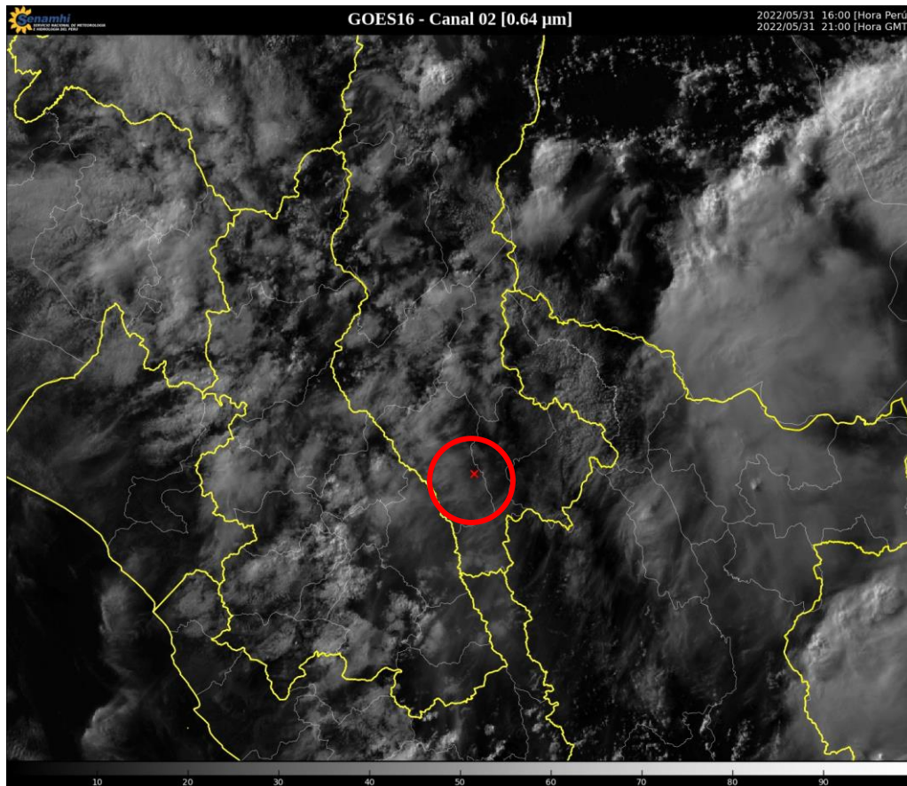
Figura 1: Imagen de Satélite GOES16 en el Canal visible del 31 de mayo de 2022 –16:00 horas.
