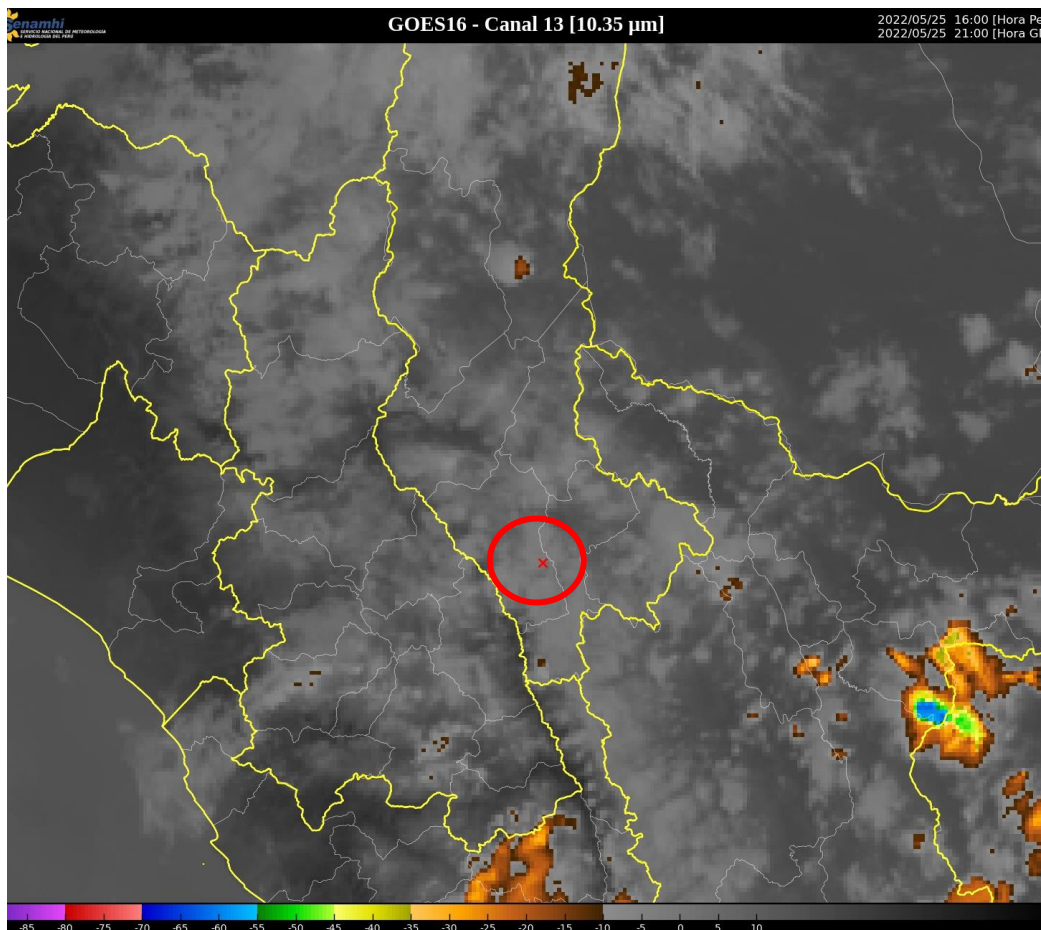
Figura 1: Imagen de Satélite GOES16 en el Canal Infrarrojo del 25 de mayo de 2022 –16:00 horas.
