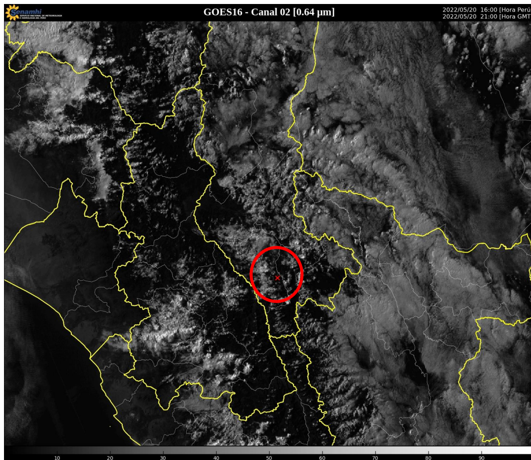
Figura 1: Imagen de Satélite GOES16 en el Canal Infrarrojo del 20 de mayo de 2022 –16:00 horas.
