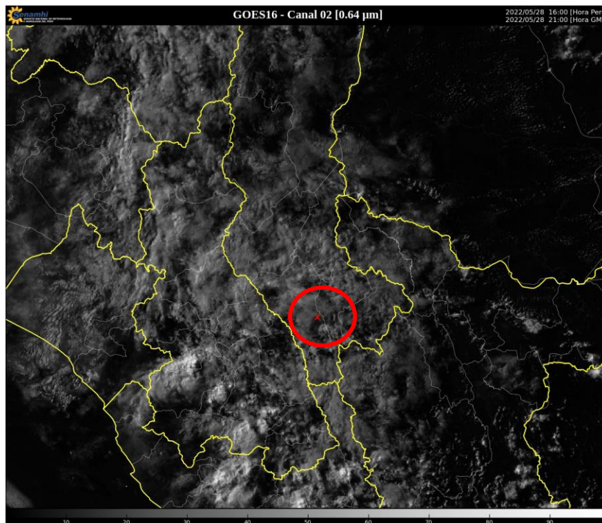
Figura 1: Imagen de Satélite GOES16 en el Canal Infrarrojo del 28 de mayo de 2022 –16:00 horas.
