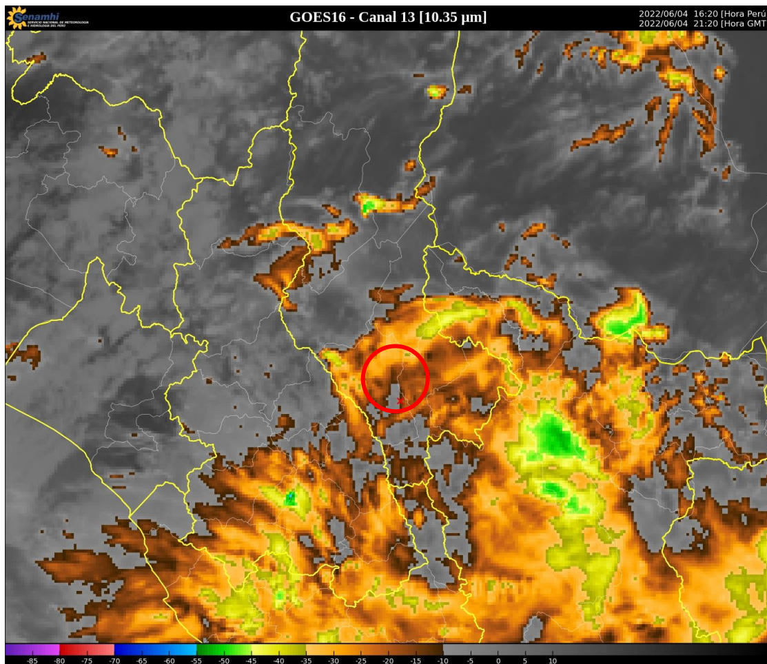
Figura 1: Imagen de Satélite GOES16 en el Canal infrarrojo del 04 de junio de 2022 –16:20 horas.
