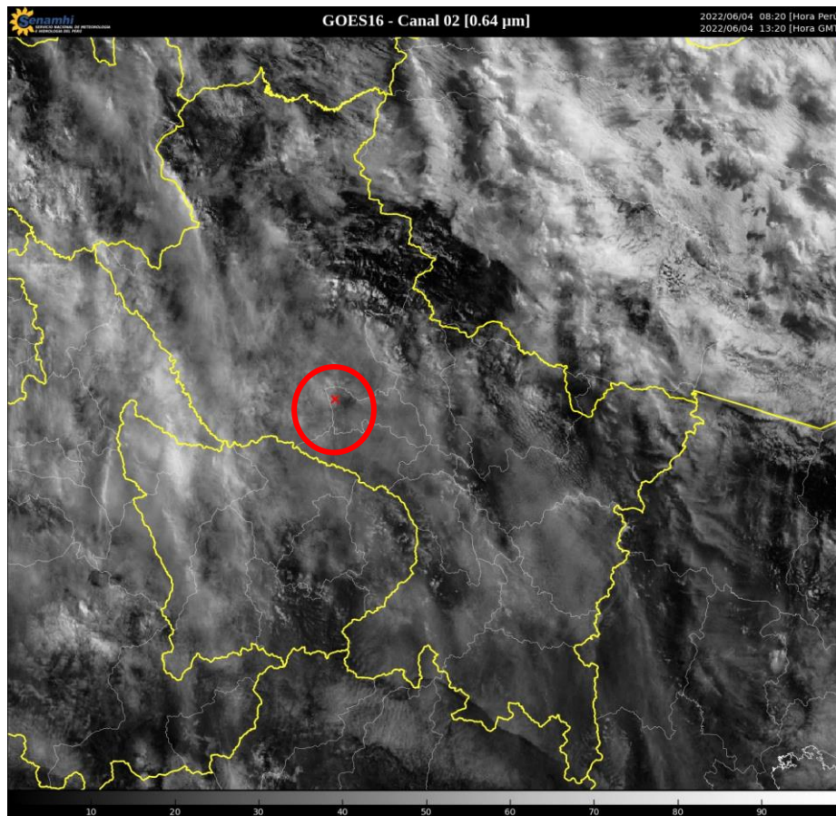
Figura 1: Imagen de Satélite GOES16 en el Canal visible del 04 junio de 2022 08:20 horas.
