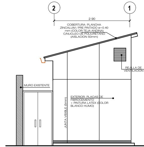
ELEVACION LATERAL Esc. 1/50
