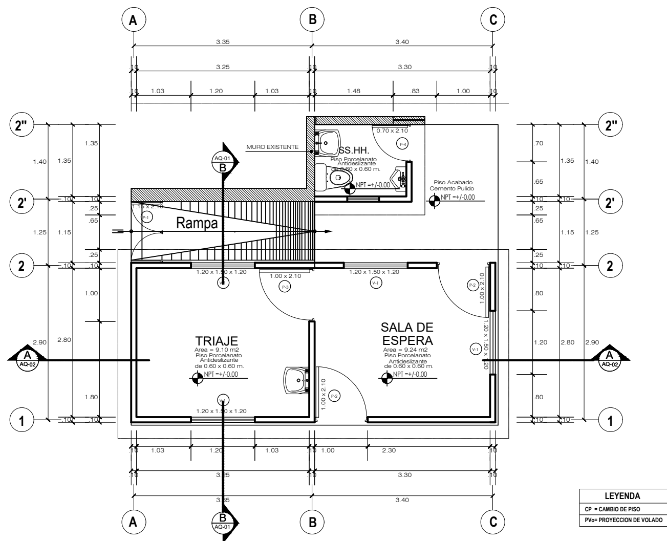
DISTRIBUCION EN PLANTA Esc. 1/50
