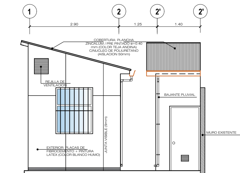
ELEVACION LATERAL Esc. 1/50
