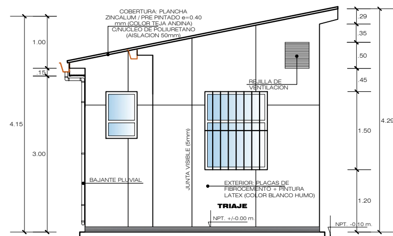
ELEVACION POSTERIOR
