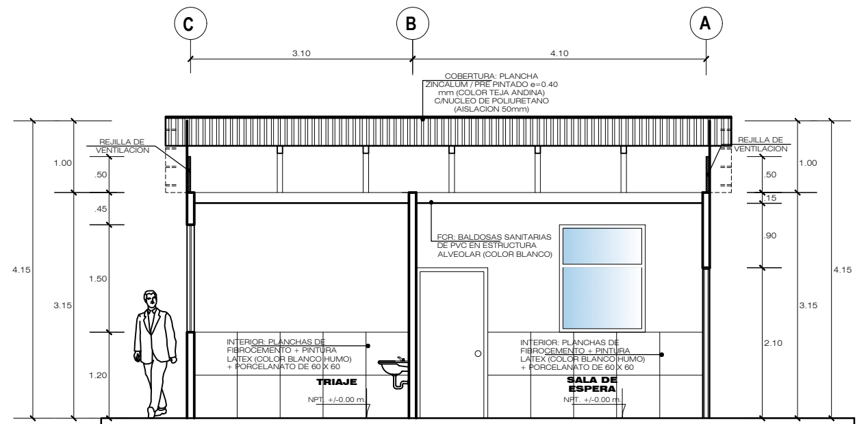
SECCION A - A
