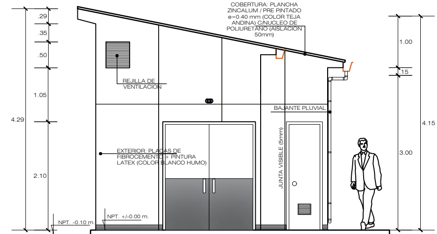
ELEVACION FRONTAL
