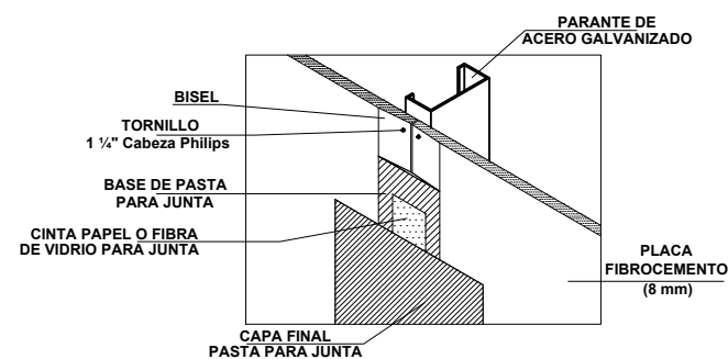
DETALLE DE UNION Esc. S/E
