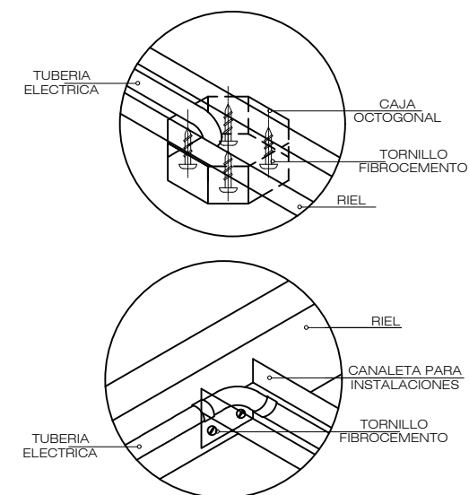
DETALLES DE ISOMETRICO Esc. S/E
