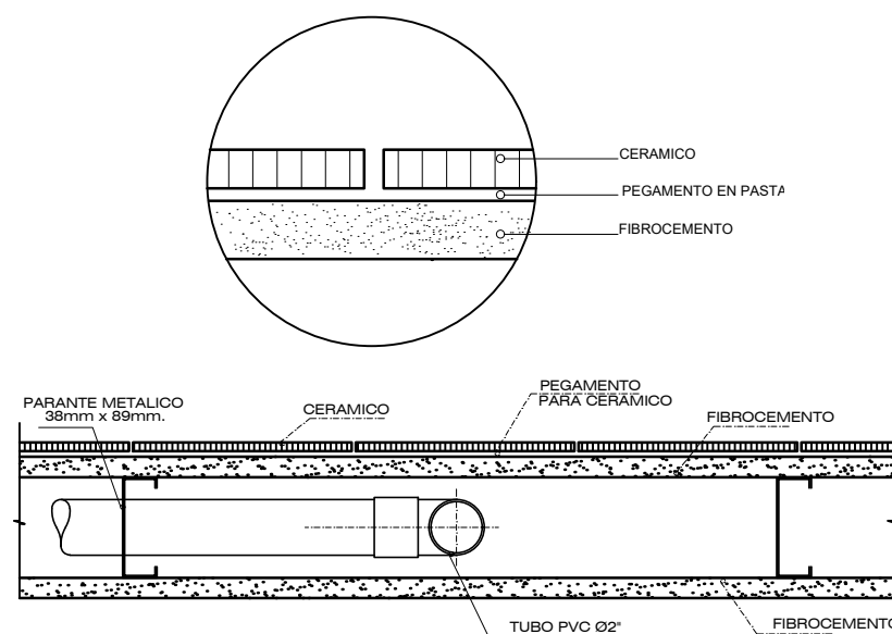
DETALLE DE ENCUENTRO / TABIQUE Esc. S/E
