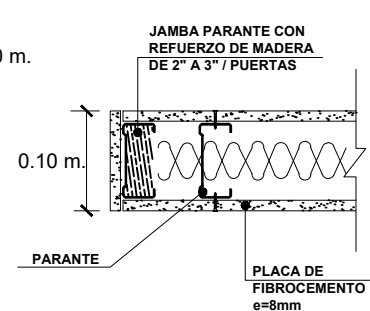
JAMBA DE MUROS Esc. 1/20
