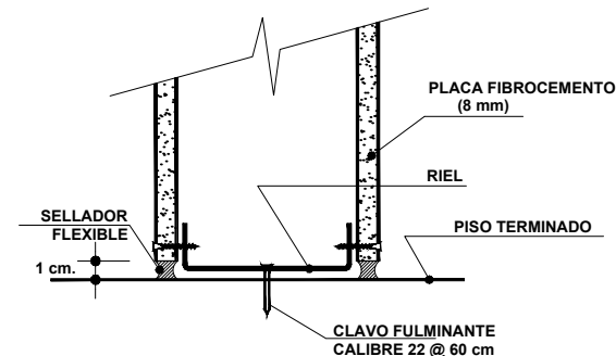
DETALLE DE ENCUENTRO / PISO Esc. 1/10
