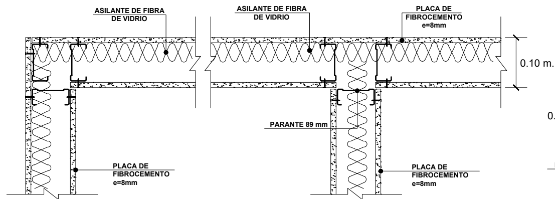
ENCUENTRO EN "L" Esc. 1/20
