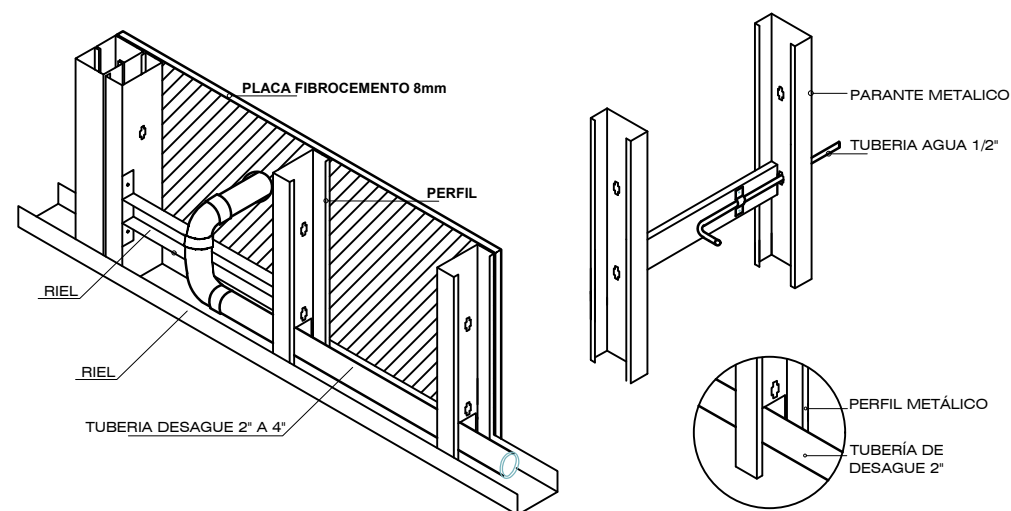
DETALLE DE INST. SANITARIAS Esc. 1/20
