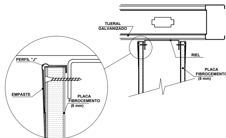
DETALLE DE ENCUENTRO / TABIQUE Esc. S/E
