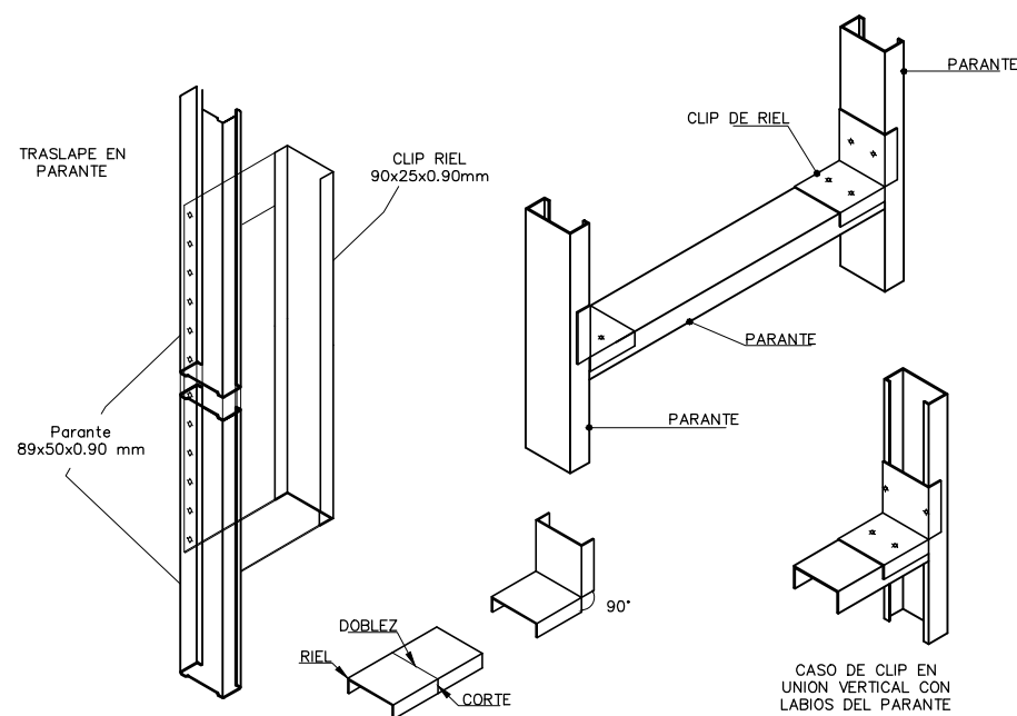
DETALLE DE EMPALME HORIZONTAL Esc. S/E
