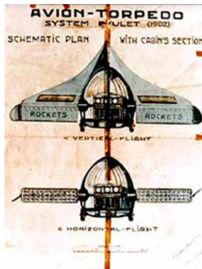
Avión torpedo diseñado por Paulet, 1902
