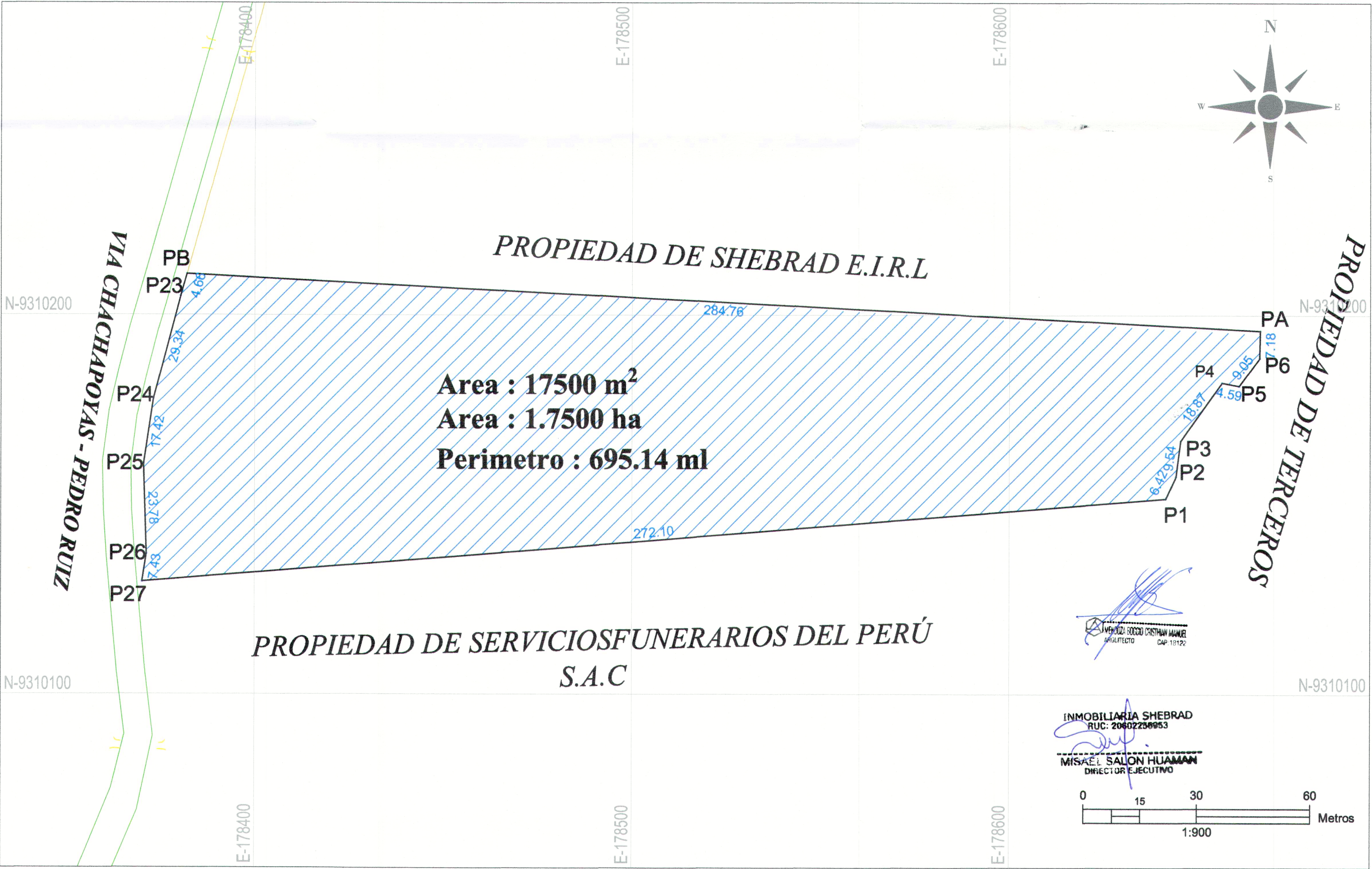
PLANO PERIMÉTRICO
