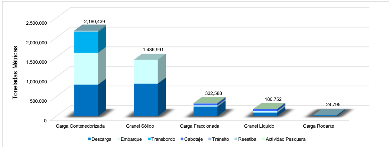
Gráfico N°1 Movimiento de carga en los terminales portuarios de uso público, según tipo de mercancía y tipo de operación, Noviembre 2022
