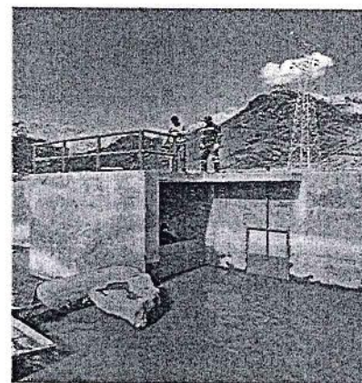
Loza de maniobra de bocatoma del Sistema de Riego Sucre
