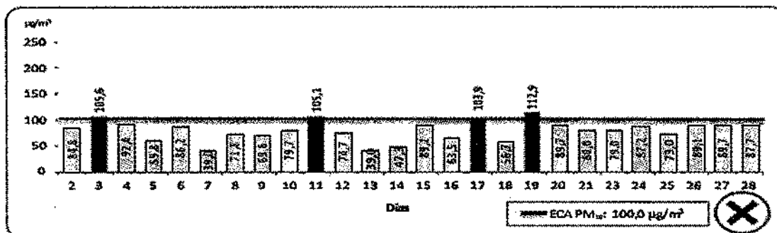
GRAFICO N° 15. LIMA ESTE. CONCENTRACION DIARIA DE MATERIAL PARTICULADO INFERIOR A 10 MICRAS, EN LA ESTACION DE MEDICIÓN DE SANTA ANITA, JUNIO 2022.
