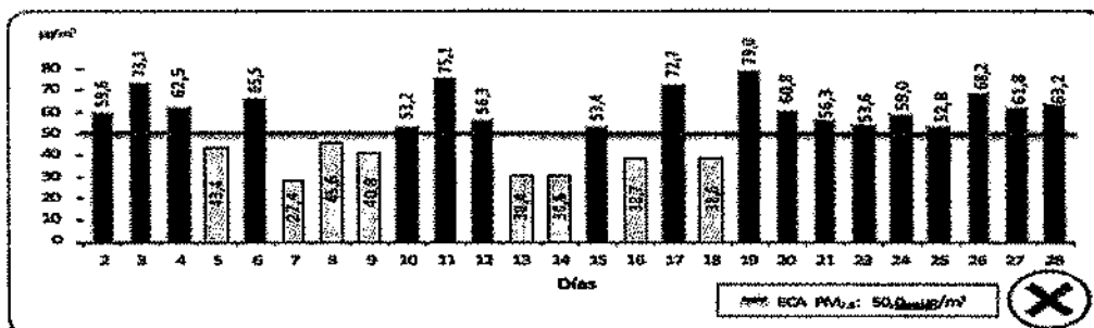
GRAFICO N° 16. LIMA ESTE. CONCENTRACION DIARIA DE MATERIAL PARTICULADO INFERIOR A 2,5 MICRAS, EN LA ESTACION DE MEDICIÓN DE SANTA ANITA, JUNIO 2022.
