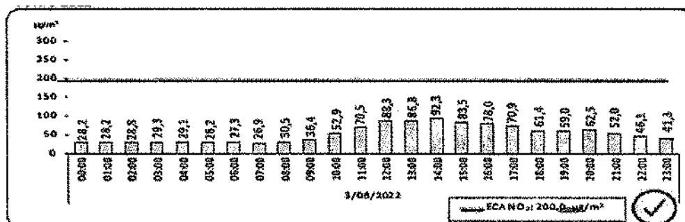
GRAFICO N° 17. LIMA METROPOLITAN: VALOR DIARIO DEL DIOXIDO DE NITROGENO (NO2), EN LA ESTACION DE SANTA ANITA, JUNIO 2022.
