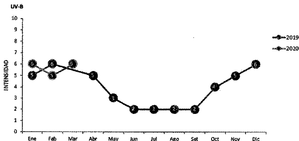
GRAFICO N° 14. LIMA. INDICE DE RADIACION ULTRAVIOLETA (IUV), SEGÚN PROMEDIO MENSUAL.
