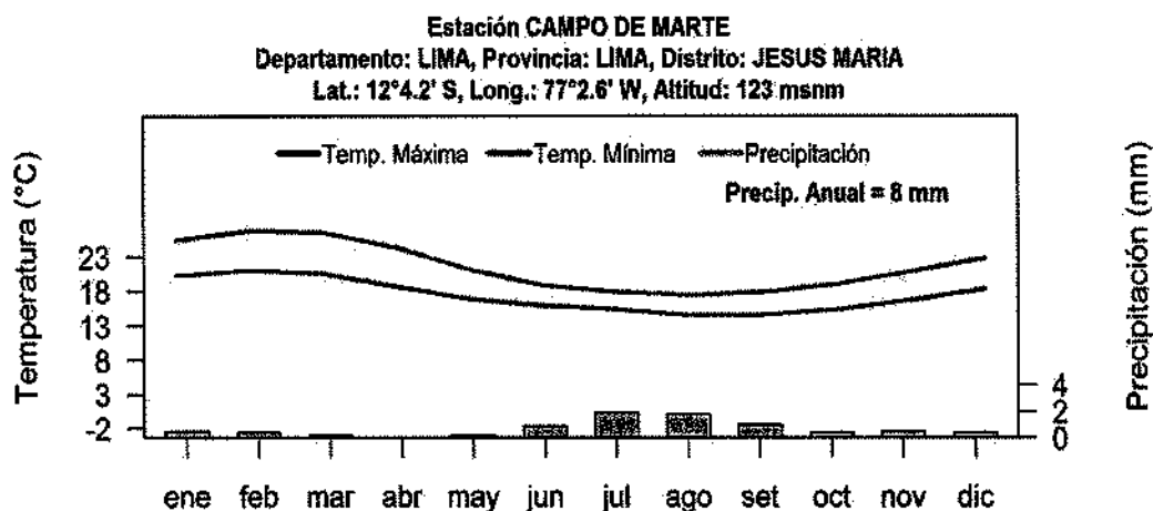
GRAFICO N° 13. DISTRIBUCIÓN TEMPORAL DE LAS TEMPERATURAS DEL AIRE Y LA PRECIPITACIÓN EN CAMPO DE MARTE.
