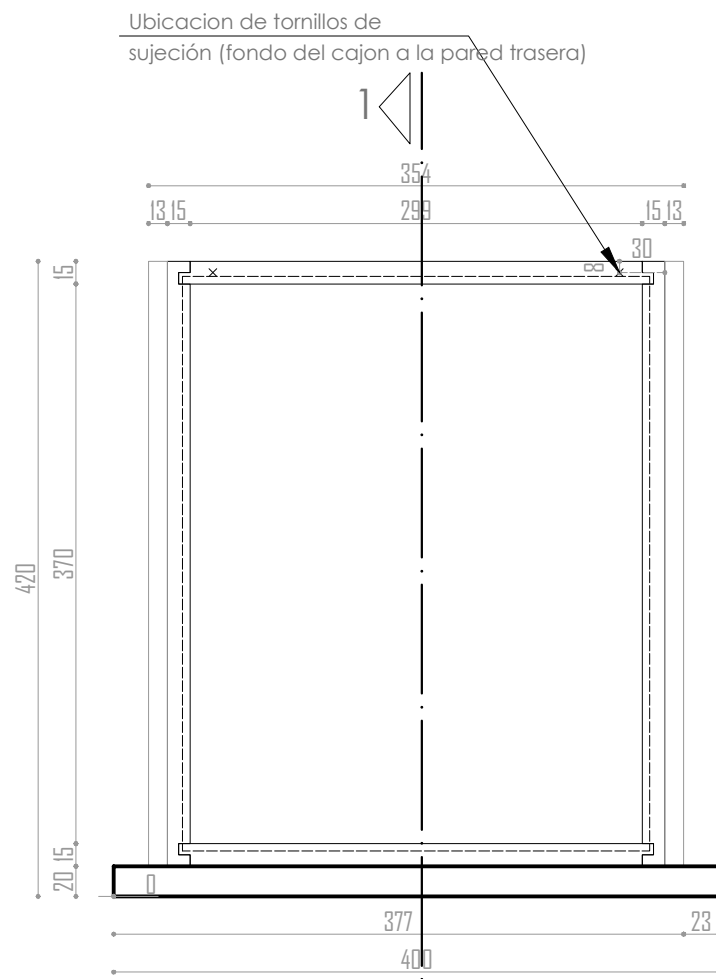
VISTA FRONTAL Escala 1 / 5
