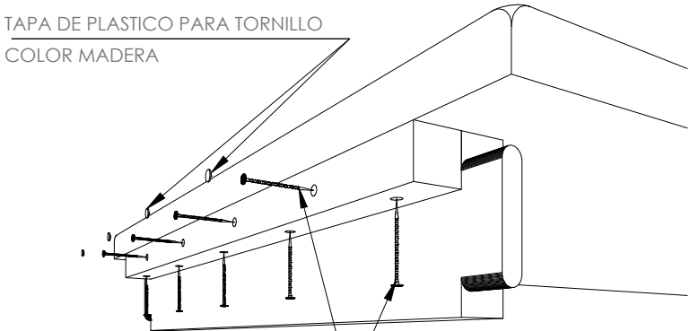
FIGURA 1 Escala 1 / 2
