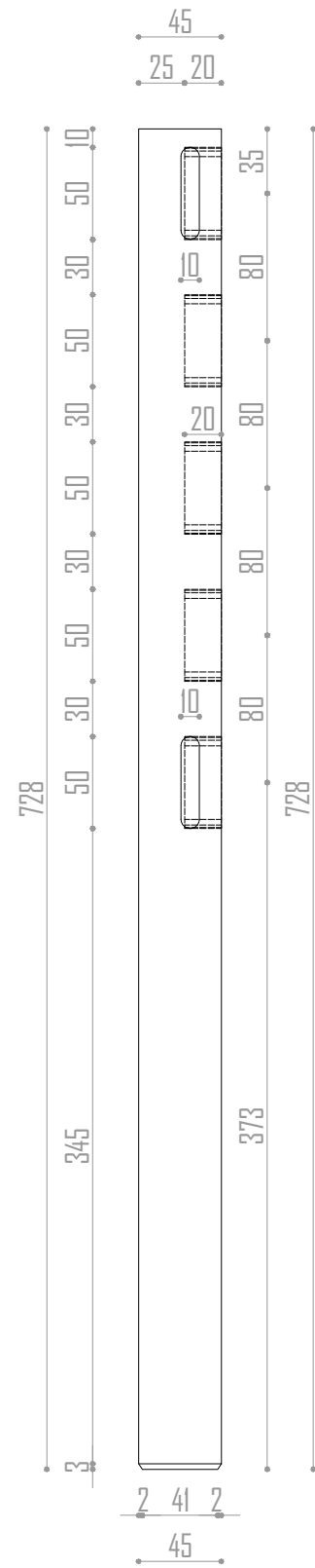
VISTA LATERAL INTERIOR Escala 1 / 4
