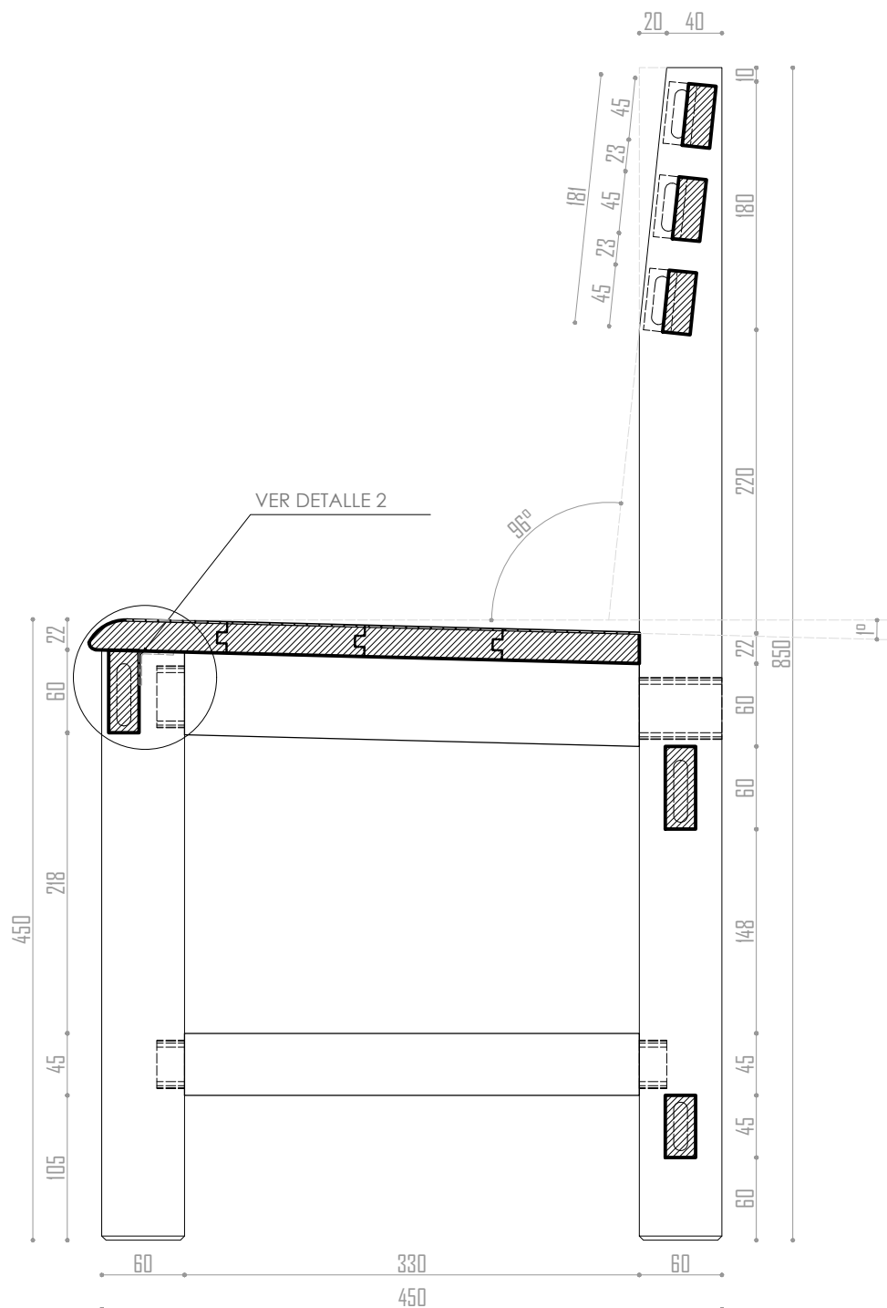
CORTE 1-1
