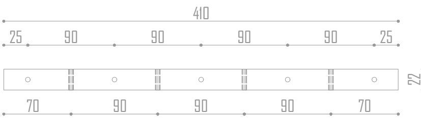
VISTA SUPERIOR Escala 1 / 4
