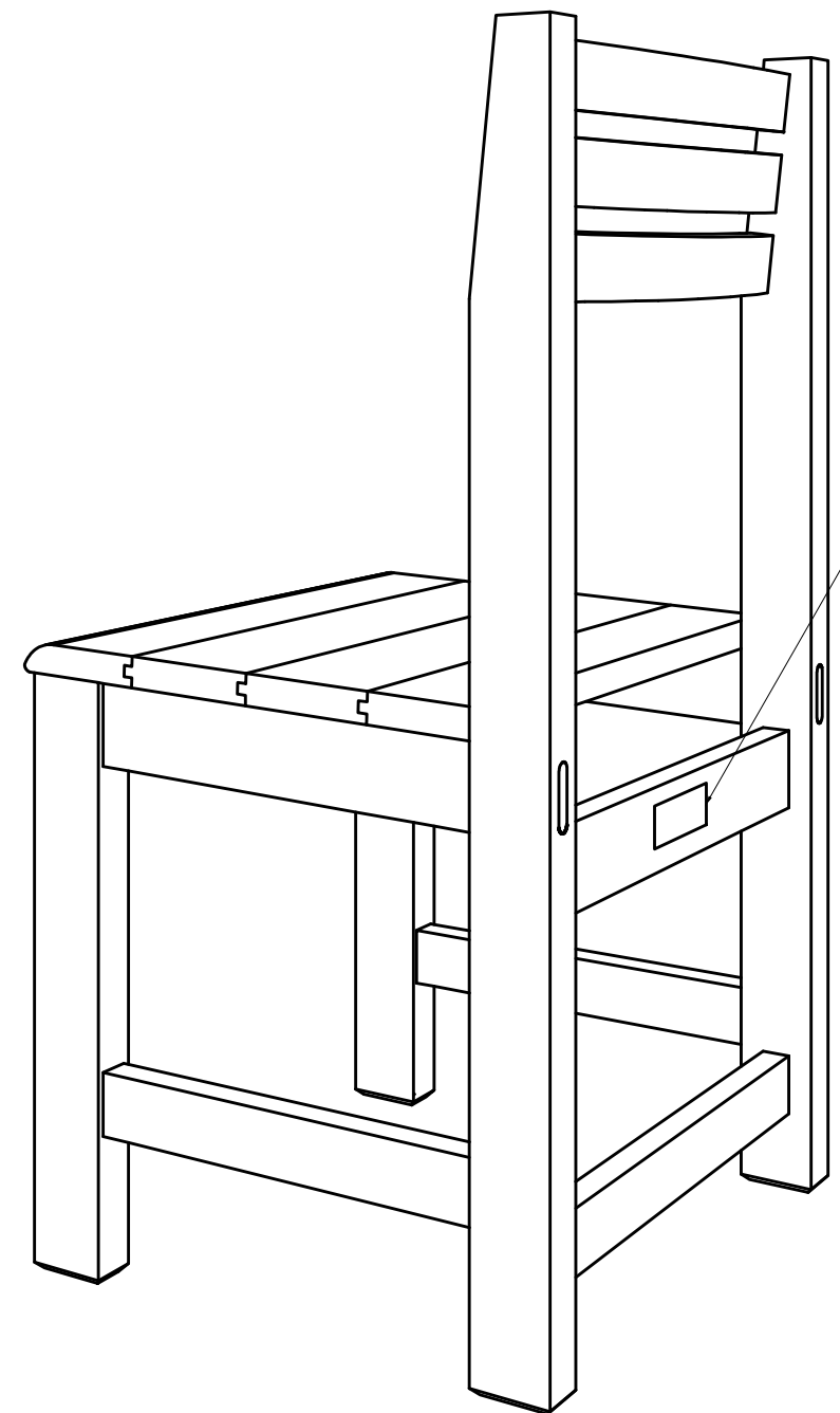
VISTA ISOMETRICA Escala 1 / 5
