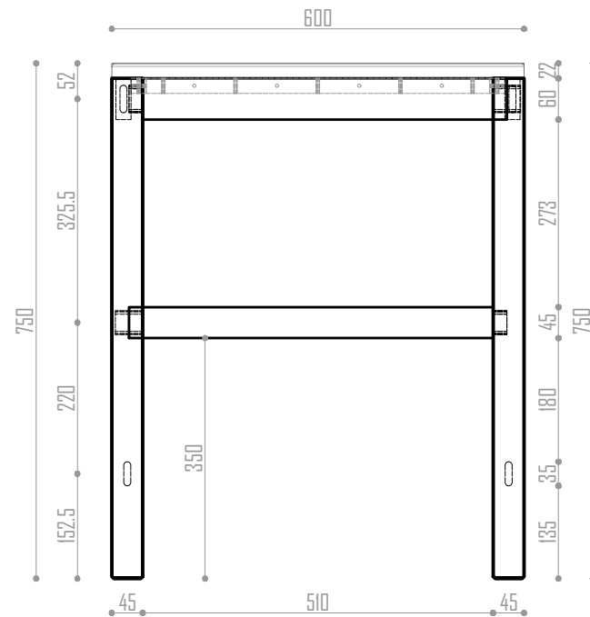
VISTA FRONTAL Escala 1 / 10
