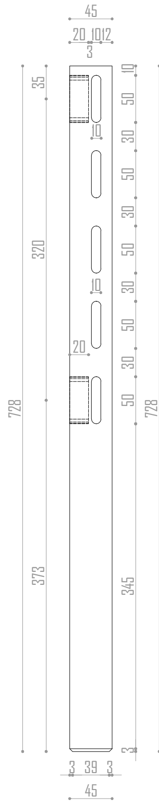
VISTA FRONTAL Escala 1 / 4
