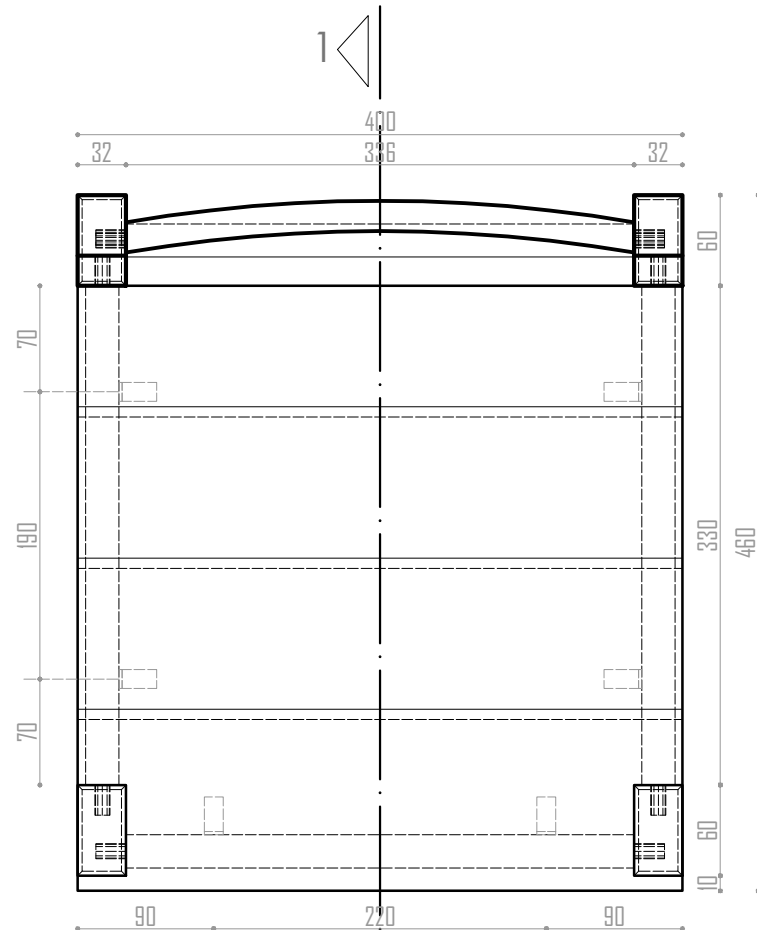
VISTA PLANTA
