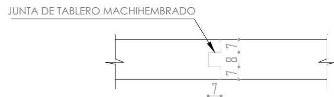
DETALLE 1 Escala 1 / 2
