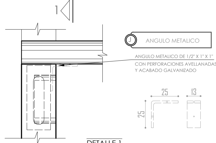
DETALLE 1
