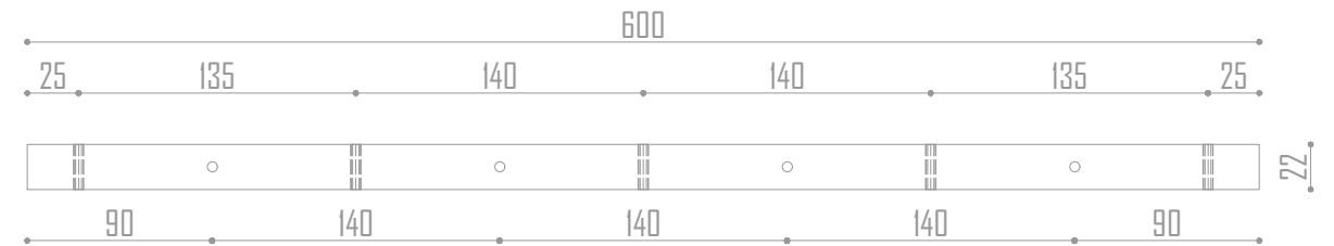
VISTA FRONTAL Escala 1 / 4
