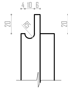
DETALLE 5 Escala 1 / 2
