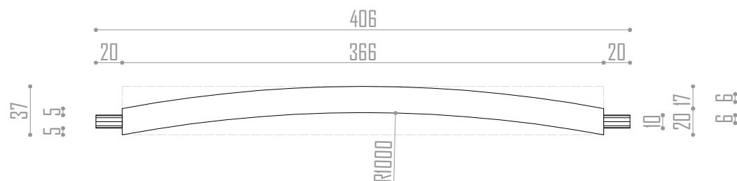
VISTA SUPERIOR
