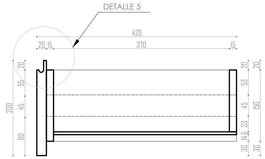
CORTE 1-1 Escala 1 / 5
