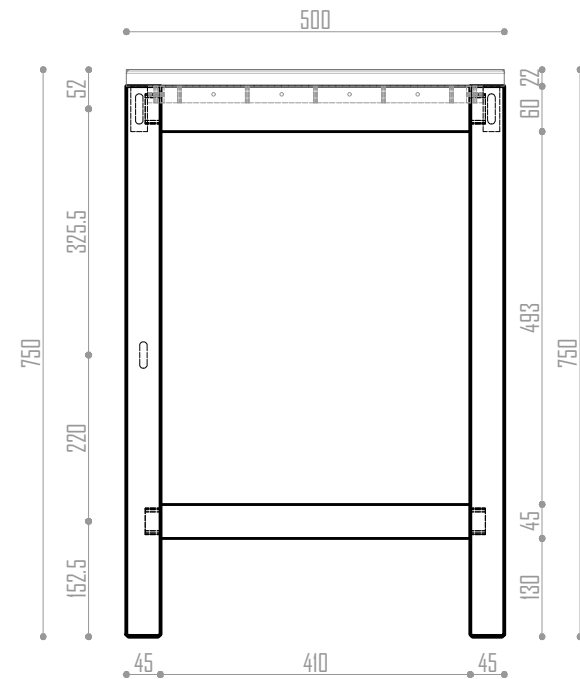
VISTA LATERAL Escala 1 / 10
