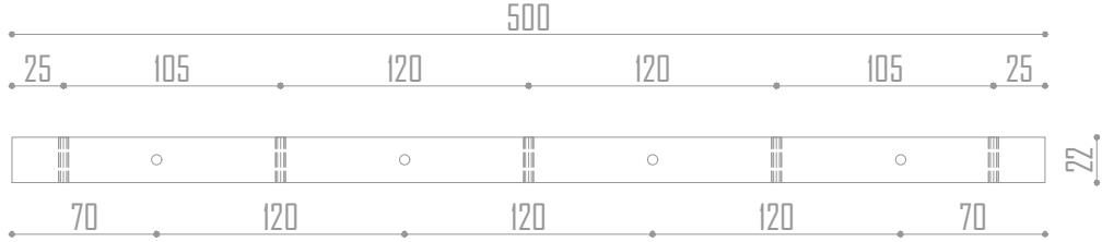
VISTA FRONTAL Escala 1 / 4
