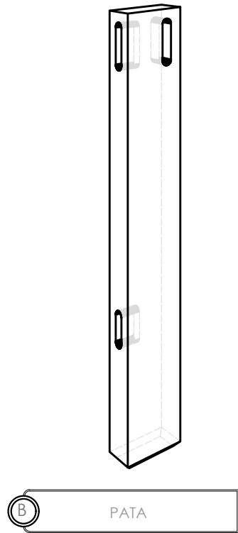
VISTA ISOMETRICA
