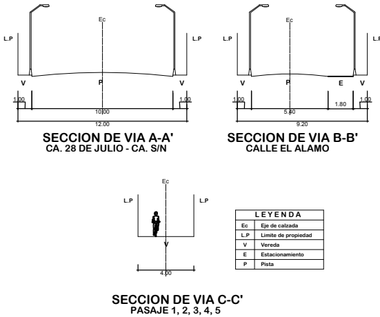
SECCIONES VIALES ESCALA: 1/200
