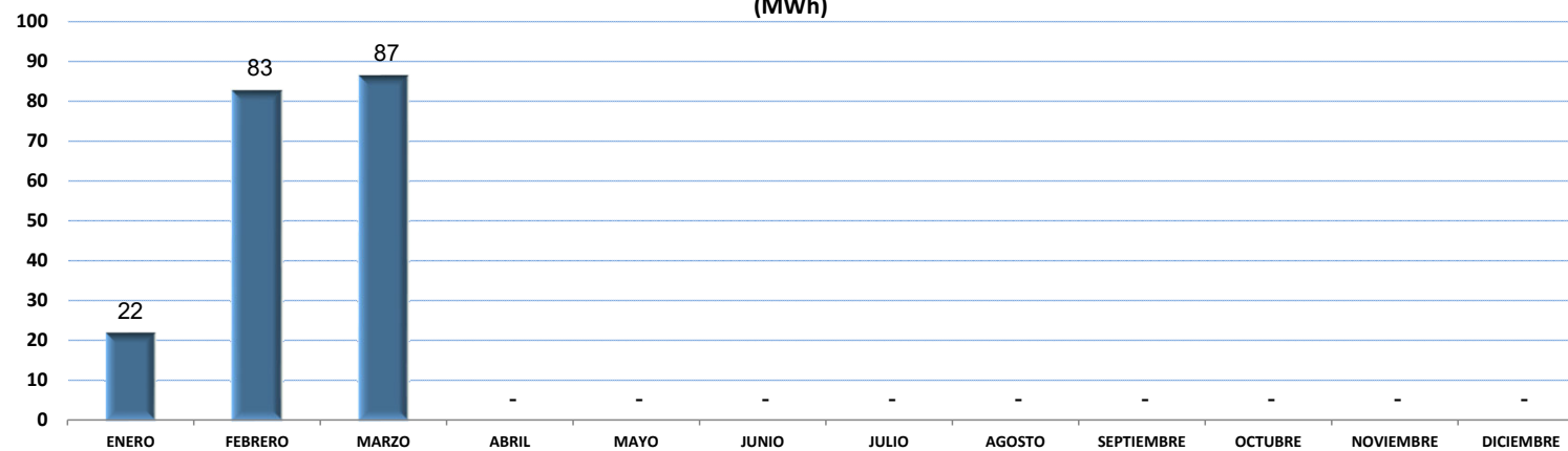
Producción de Energía Térmica - Año 2025 (MWh)
