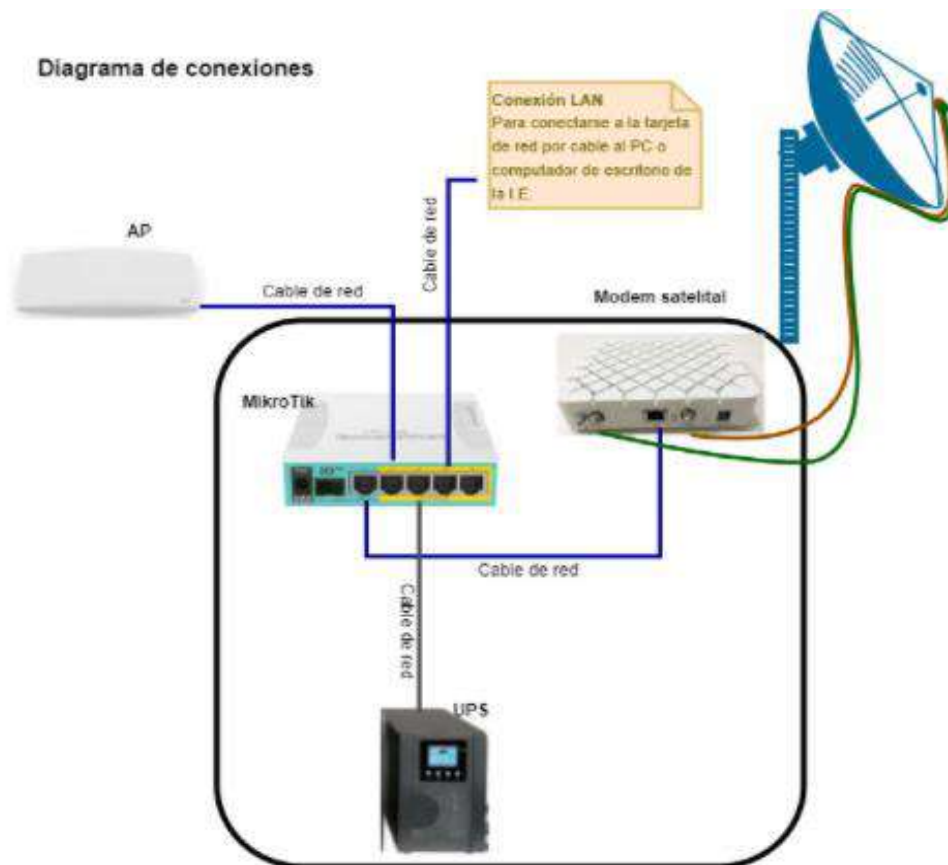
Diagrama 1. Diagrama de referencia para las conexiones equipos de cada Institución Educativa
