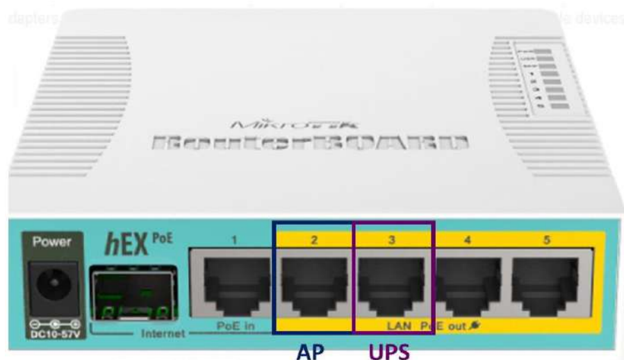
Ilustración 4. Imagen de referencia conexión AP y Ups en router de red - MikroTik
