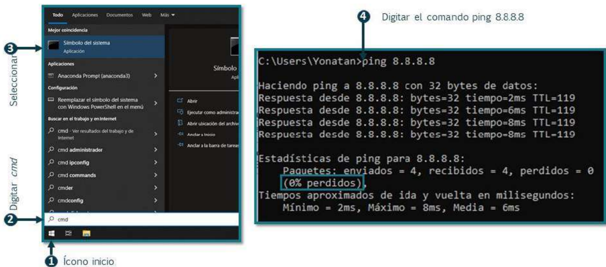
Ilustración 18. Imagen de referencia acceso a Símbolo de sistema y ejecución prueba de ping a DNS Google
