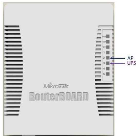
Ilustración 5. Imagen de referencia revisión de indicadores después de conectar el AP y la UPS en los puertos indicados del router de red - MikroTik
