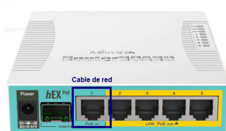
Ilustración 2. Imagen de referencia puertos router de red - MikroTik
