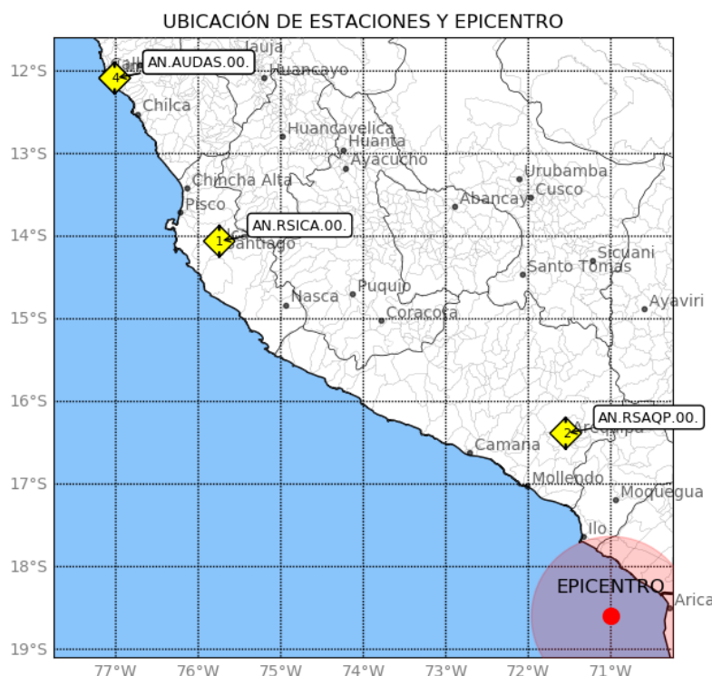
Epicentro del evento sísmico y ubicación de estaciones acelerográficas
