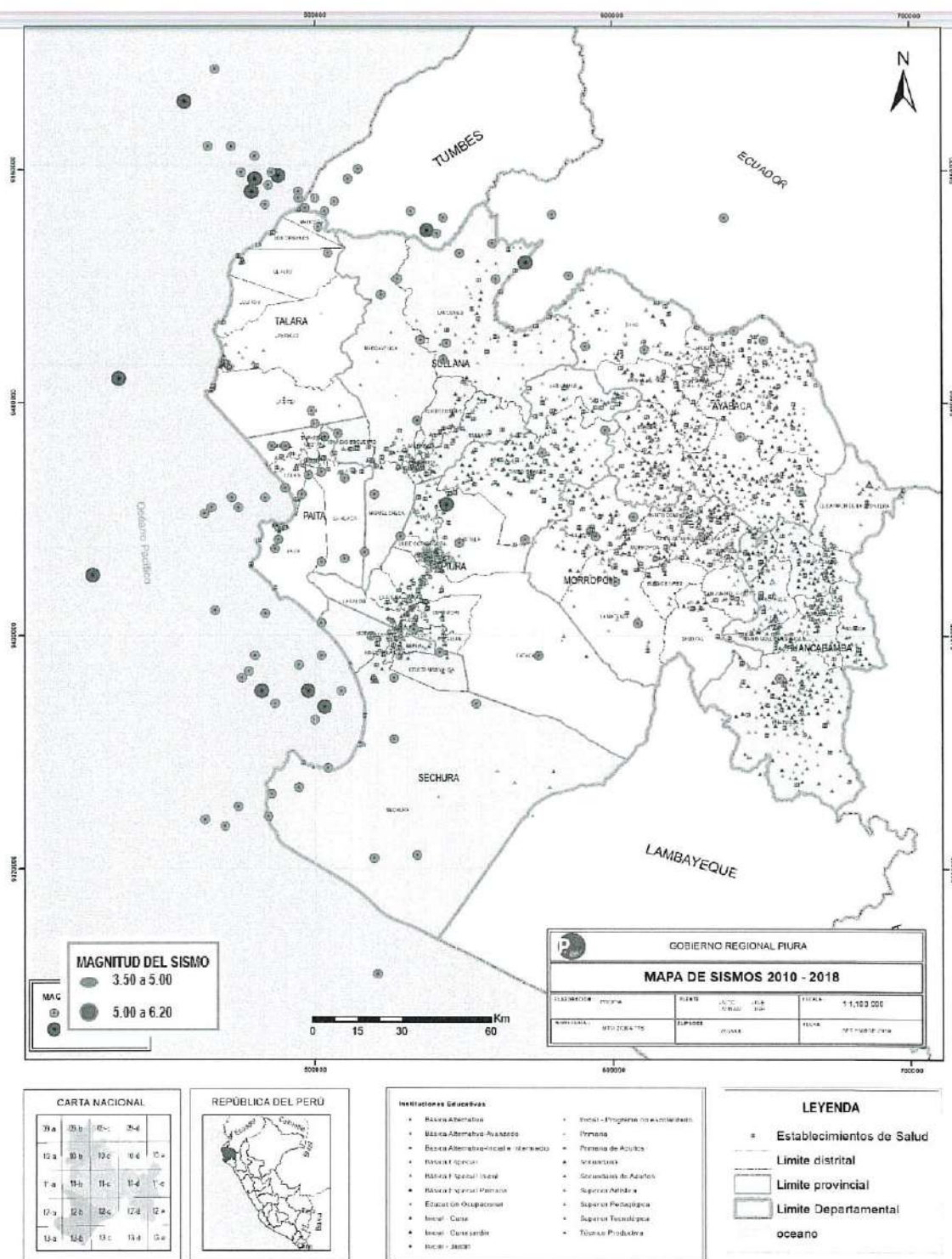
Figura 10. Mapa Sísmico de la Región Piura para el periodo 2010 y 2018.
