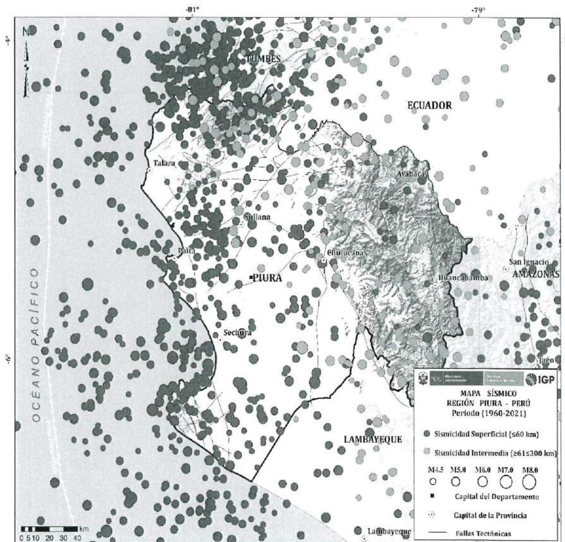
Figura 9. Mapa Sísmico de la Región Piura para el periodo 1960 y 2021.
