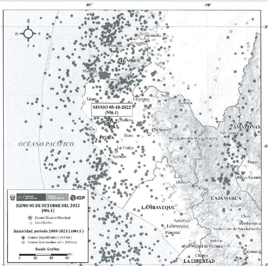
Figura 5. Mapa del sismo de 6,1 mm del 05 de octubre del 2022 – Región Piura
