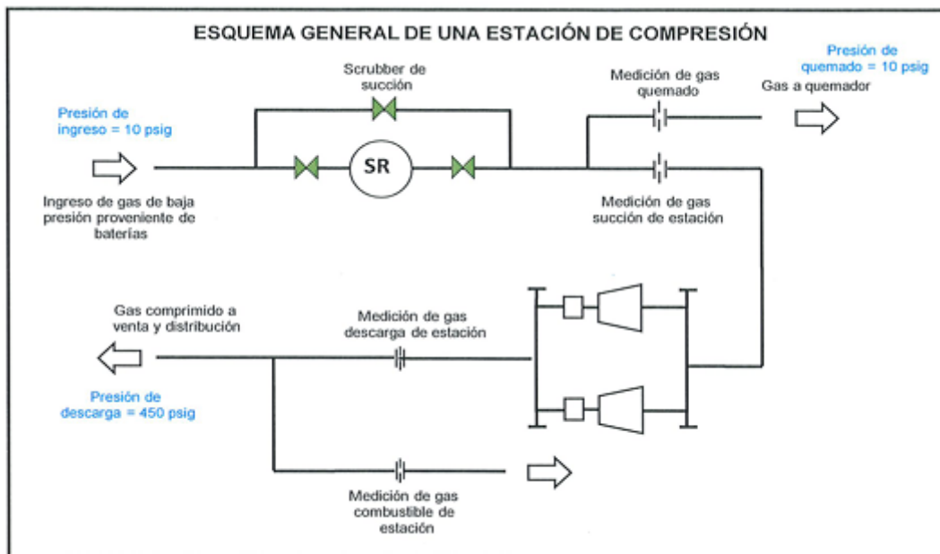
Figura N° 1: Esquema General de la Estación de Compresión – Lote X
