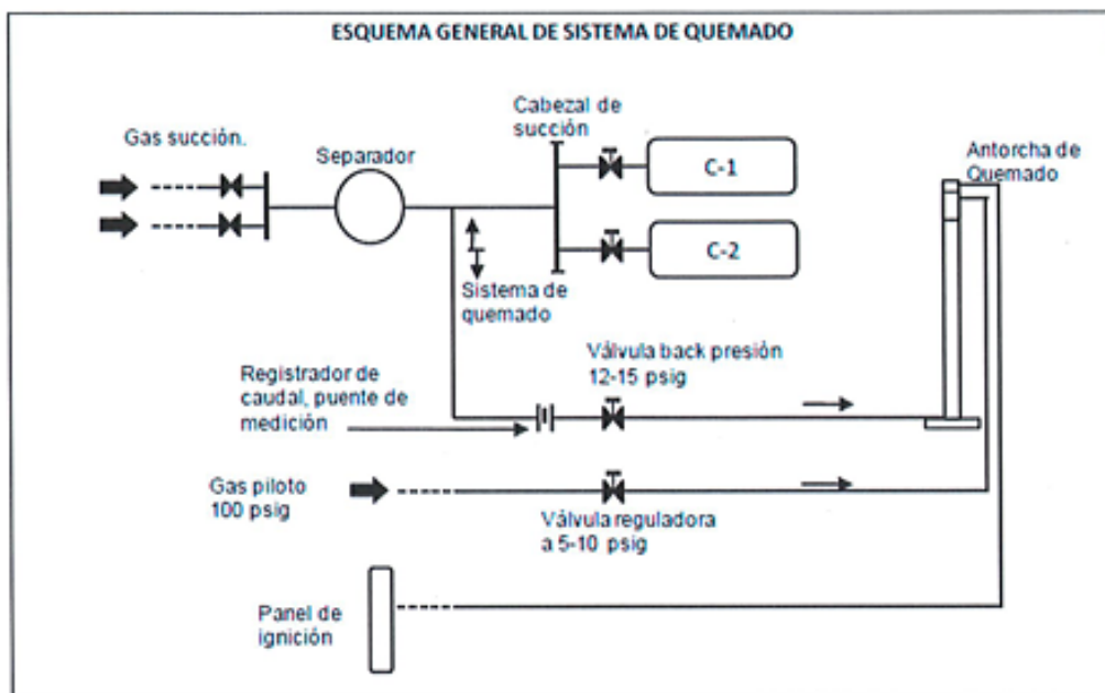
Figura N° 2: Esquema General de Sistema de Quemado – Lote X
