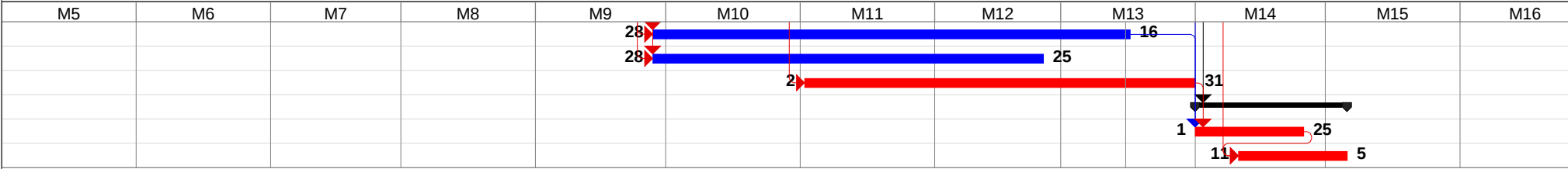
CRONOGRAMA DE OBRA LINEAS PRIMARIAS, REDES PRIMARIAS, REDES SECUNDARIAS Y CONEXIONES DOMICILIARIAS
