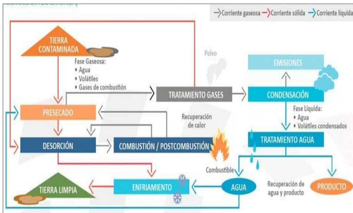
Figura 5-10 Esquema representativo de desorción térmica
