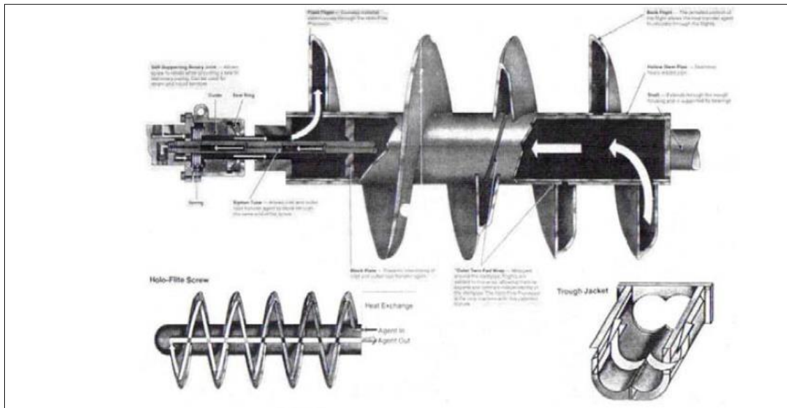
Figura 5-9 Representación de tornillo sin fin
