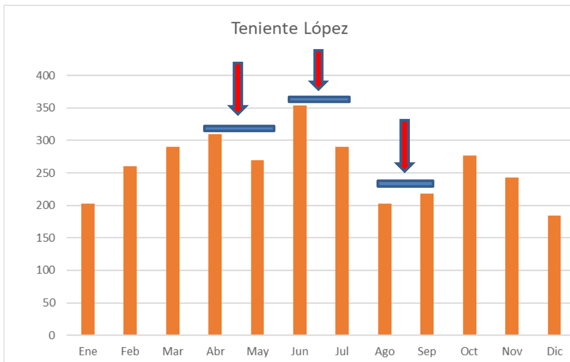
Figura 2-8 Histograma de precipitación (2000-2006) estación teniente López
