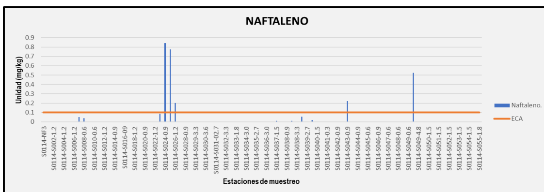
Figura 3-17 Concentraciones de naftaleno
