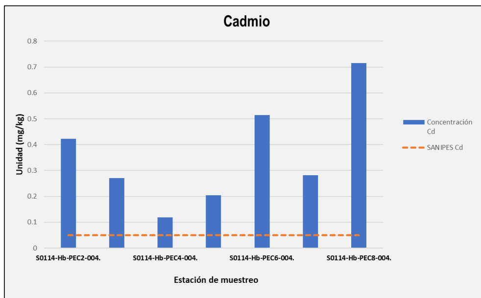
Figura 4-26 Concentraciones de Cadmio – Época seca
