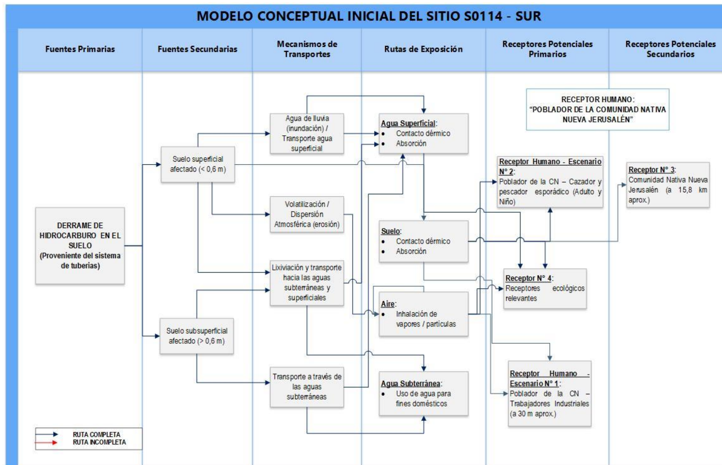
Figura 4-29 Modelo conceptual inicial del sitio S0114 (Sitio 14) – Zona Sur
