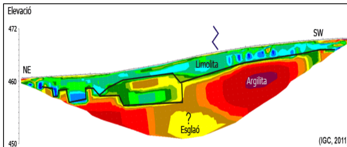
Figura 3-11 Modelo de resistividad eléctrica del subsuelo en una tomografía eléctrica
