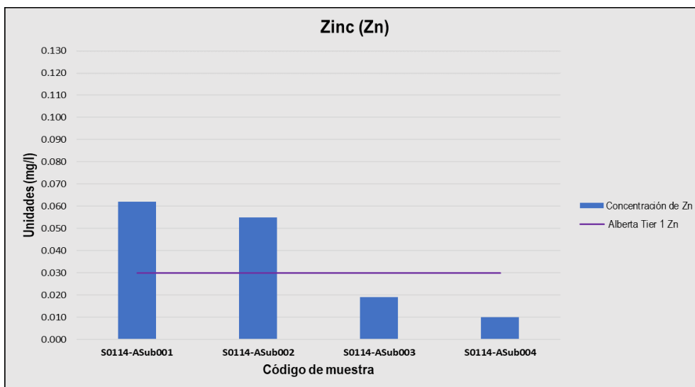
Figura 4-23 Concentraciones de Zinc – Época seca
