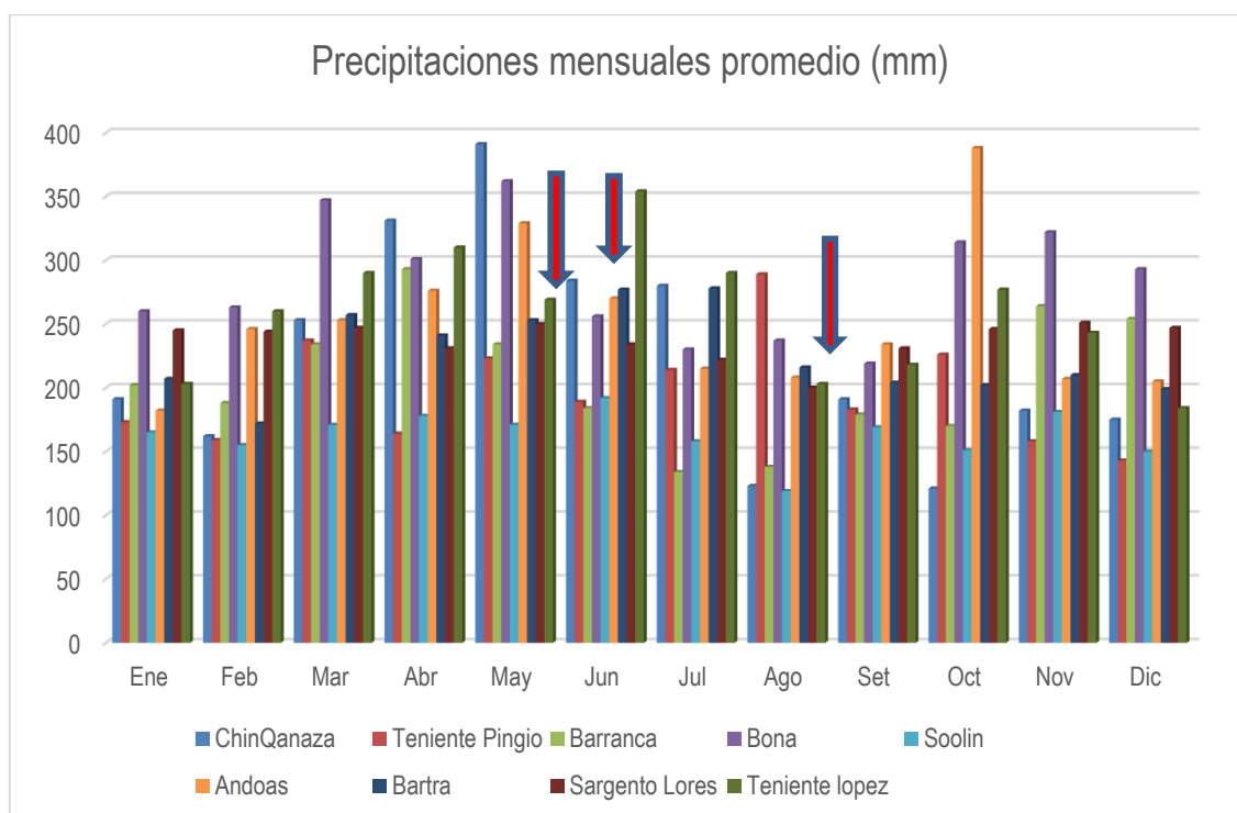
Figura 2-9 Histograma de precipitación estaciones cercanas al Lote 1AB (Ex lote 1AB) (2000-2006).
