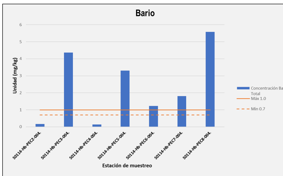
Figura 4-28 Concentraciones de Bario – Época seca
