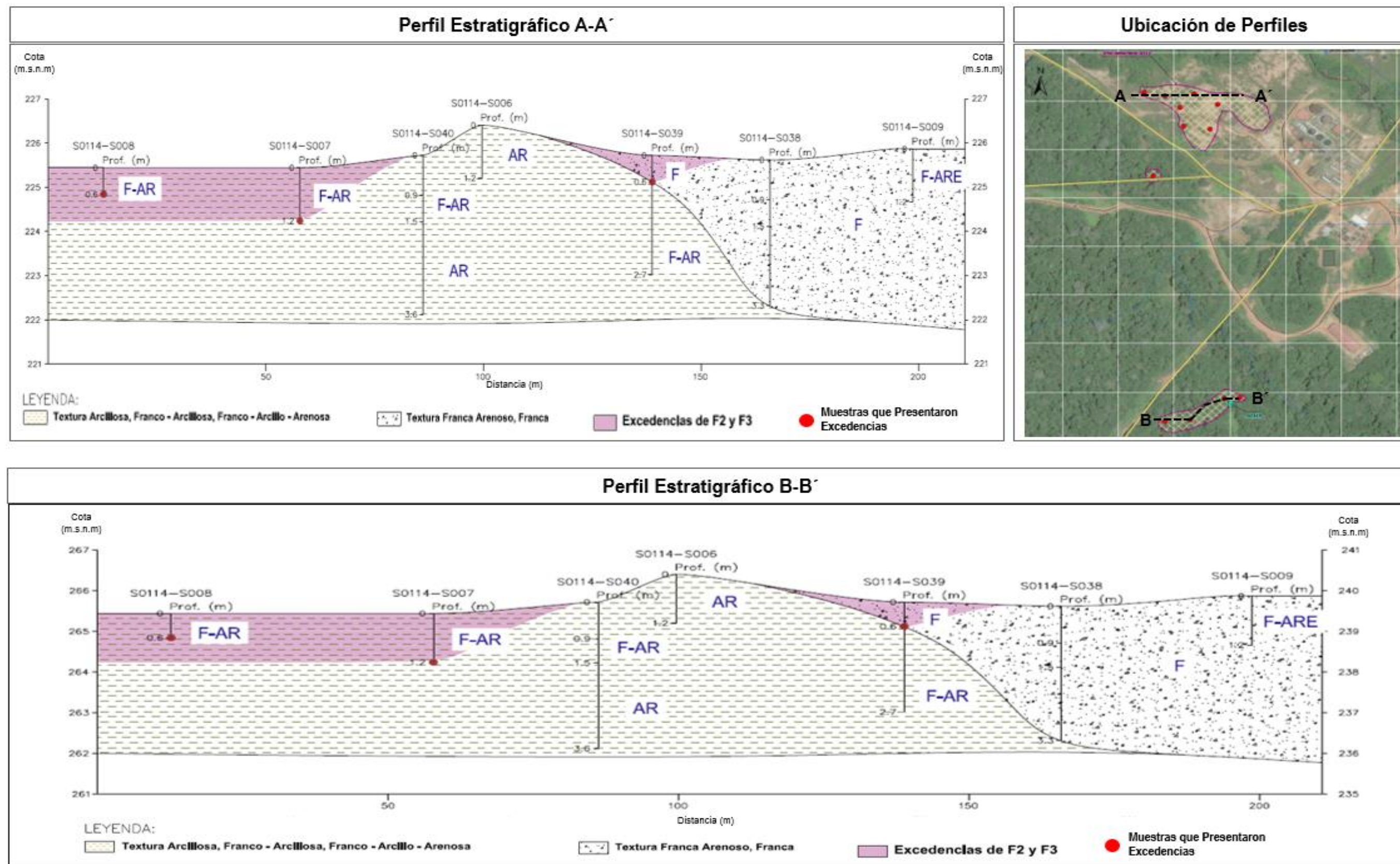
Figura 3-26 Delimitación del sitio impactado (Fracción integrada de hidrocarburos F2 y F3)
