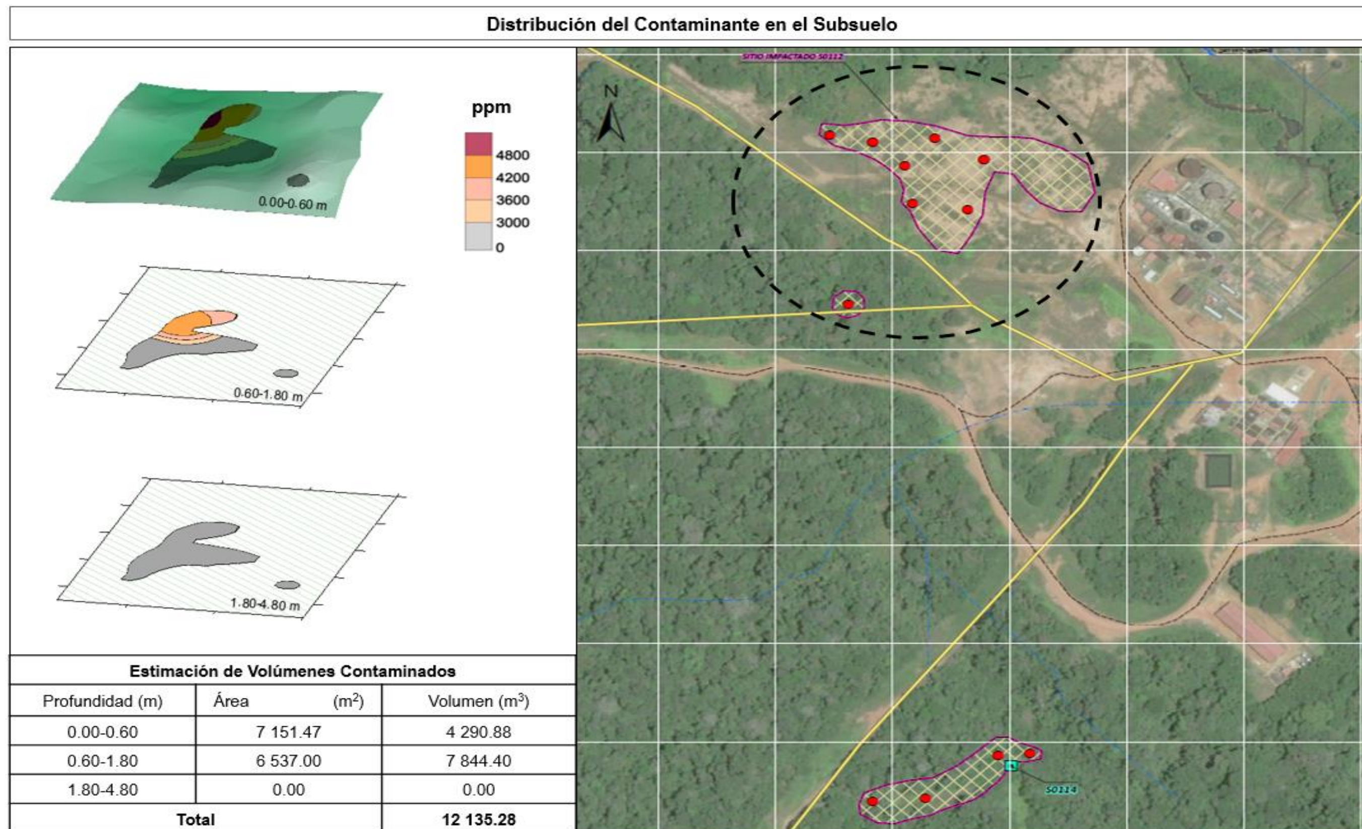
Figura 3-28 Delimitación del sitio impactado (Fracción de hidrocarburos F3)
