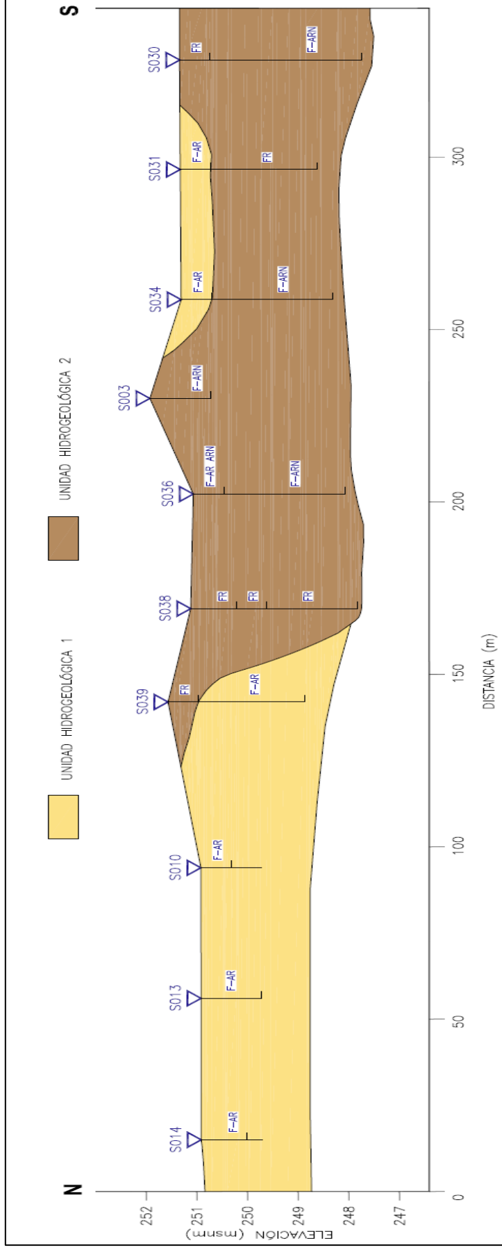
Figura 2-6 Perfil hidrogeológico del sitio S0114 (Sitio 14) al sur de la Bateria Dorissa
