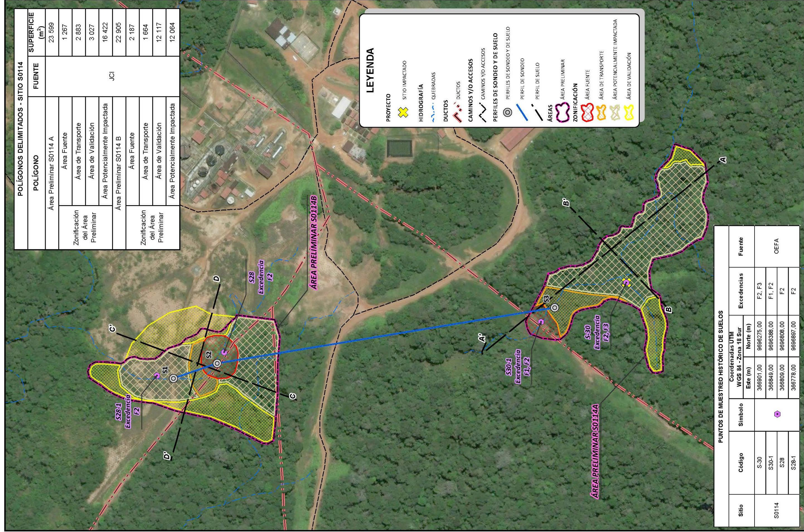
Figura 3-31 Área potencial de interés (API) de acuerdo con el MCI
