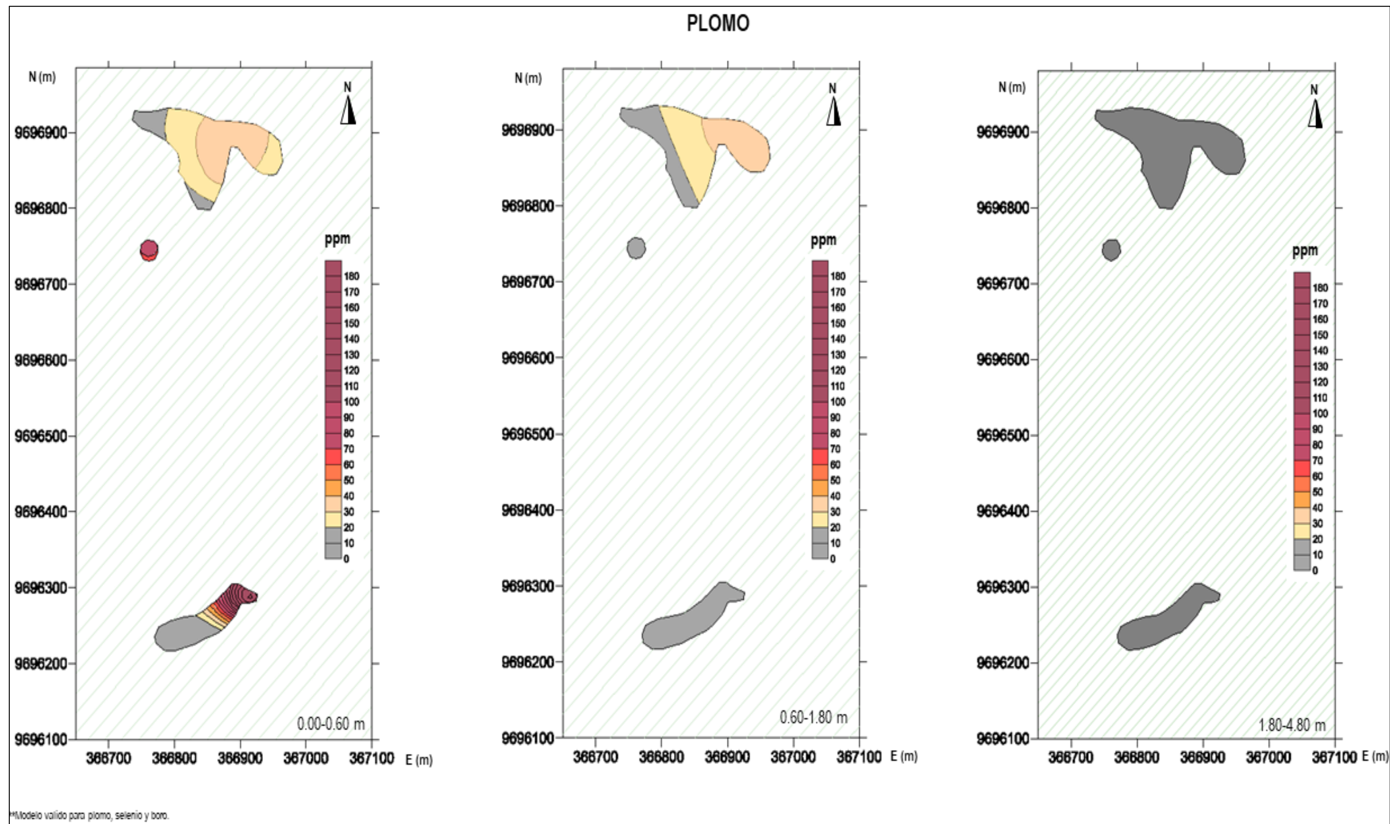
Figura 3-21 Modelamientos de Isoconcentraciones
