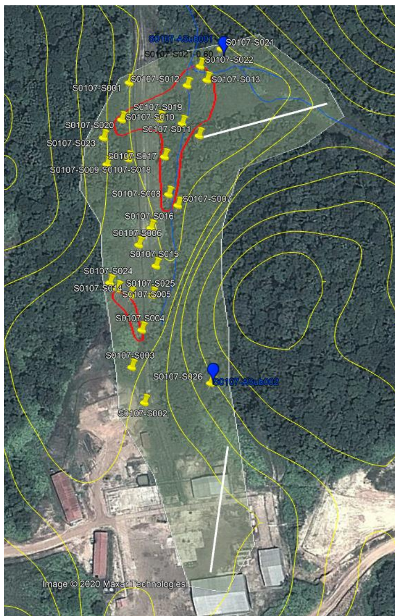
Figura 2-Ob-1c Delimitación del área de evaluación geológica-hidrogeológica
