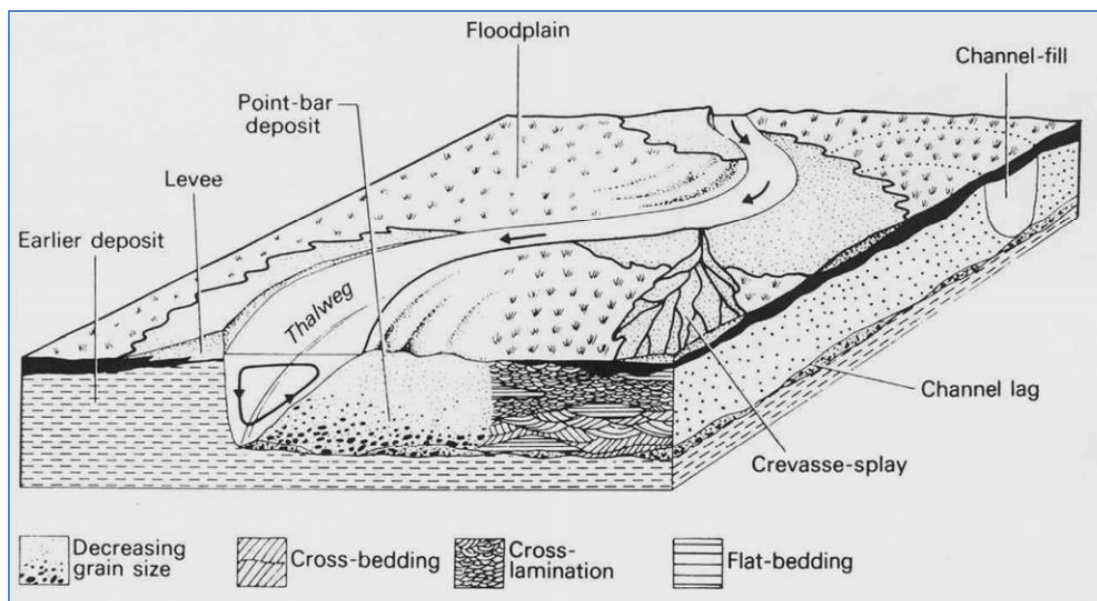
Figura 0-Ob-1b Modelo de ambientes de sedimentación (ríos meandriformes)
