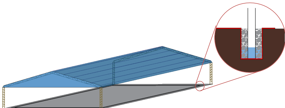
Figura 5-13 Área de almacenamiento provisional
