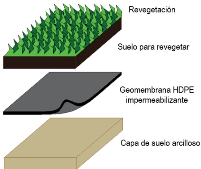
Figura 5-15 Estructura de cierre del área de aislamiento
