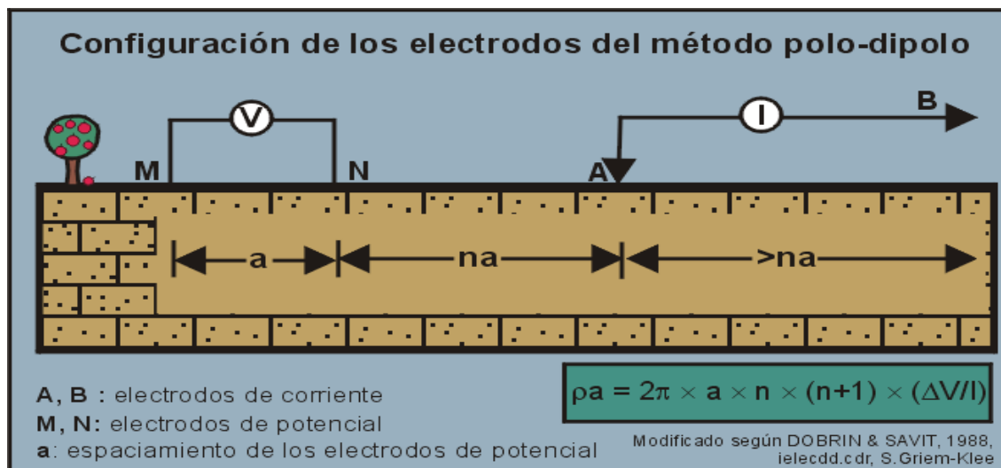
Figura 3-10 Configuración de los electrodos del arreglo polo-dipolo
