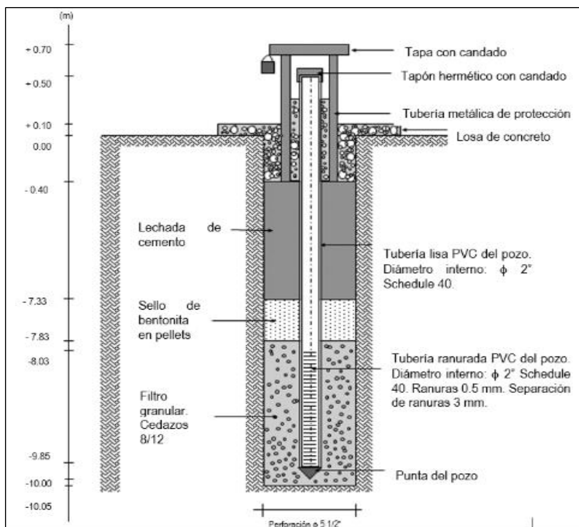
Figura 3-9 Detalles constructivos típicos de terminación de pozos
