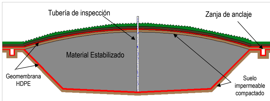
Figura 5-16 Sección esquemática de la topografía final del espacio de aislamiento después del cierre
