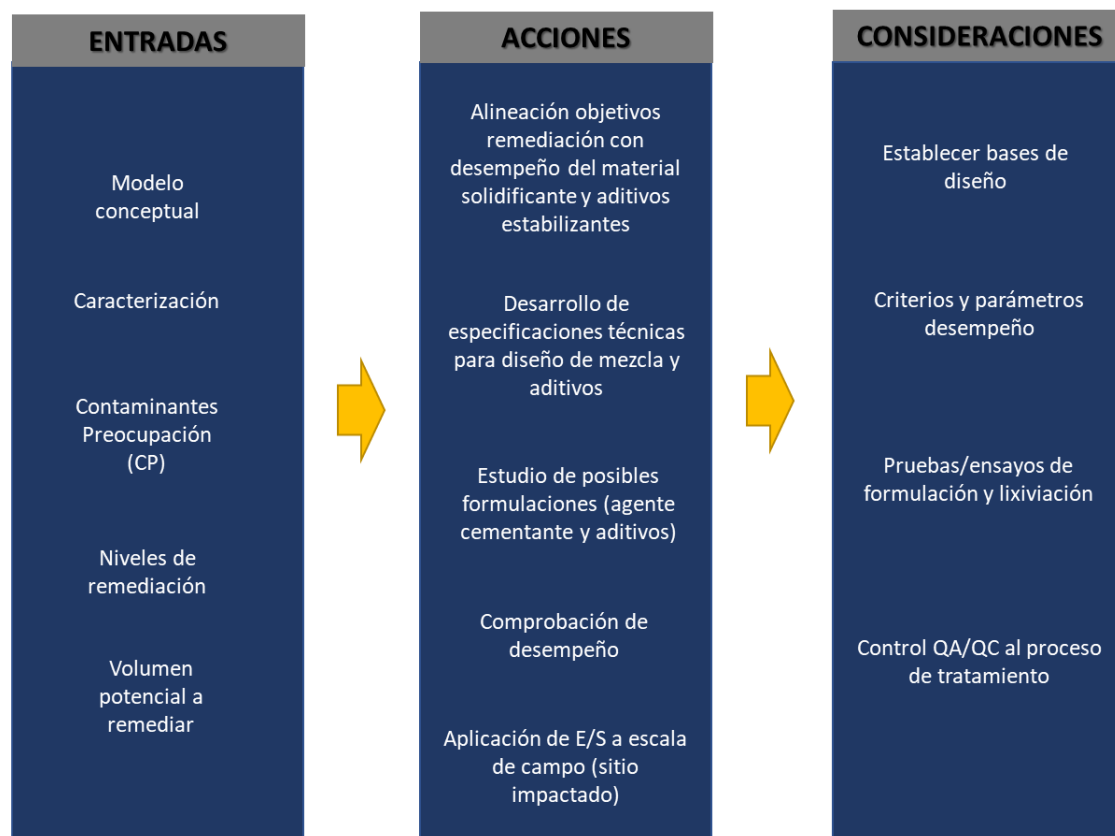
Figura 5-9 Etapas para la planificación de la estabilización/solidificación
