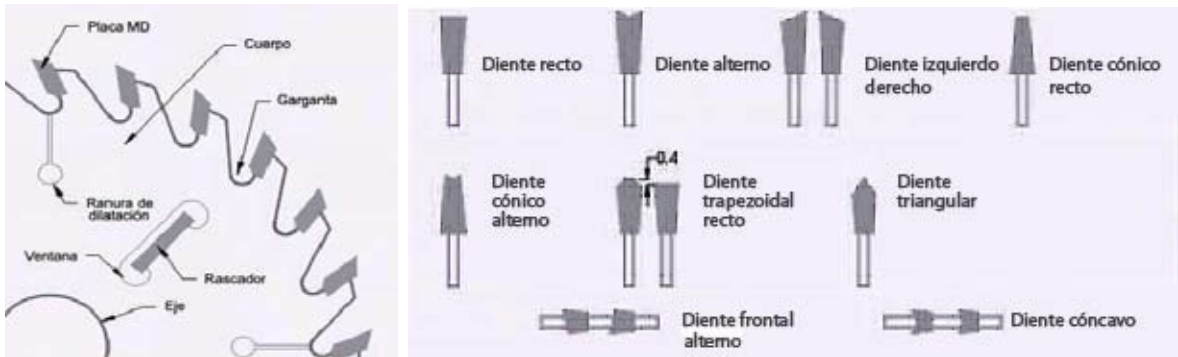
Gráfico 8. Disco y tipos de dientes de las sierras
