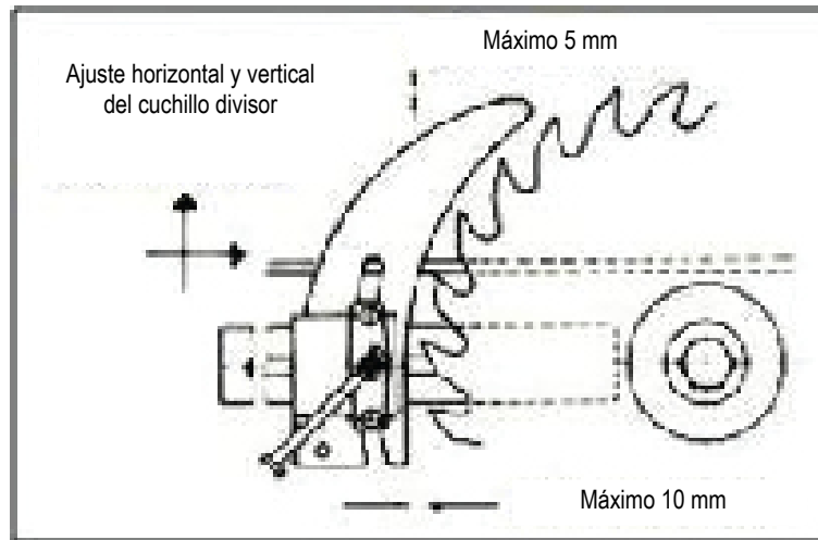
Grafico 11. Ajuste horizontal y vertical del cuchillo divisor
