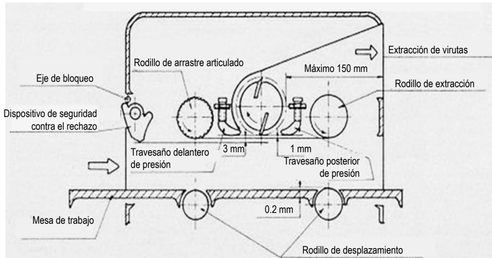
Grafico 14. Partes de la cepilladora o regruesadora
