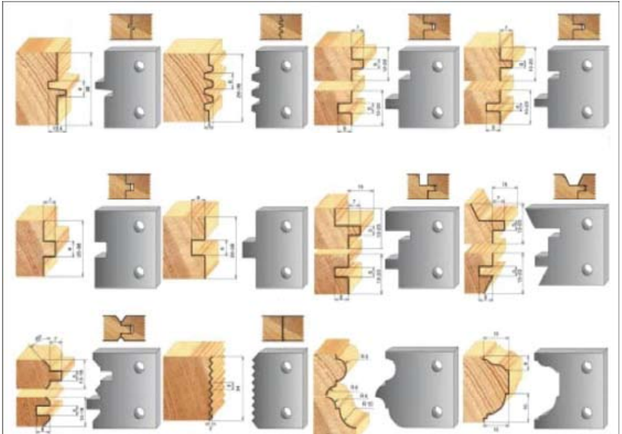
Grafico 16. Perfiles según tipos de cuchillas usadas en el cabezal porta cuchillas del Tupí
