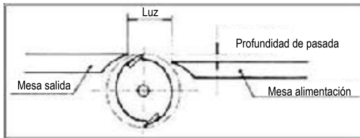
Grafico 13. Calibración de las cuchillas a nivel de la mesa de salida
