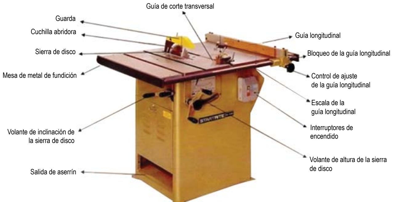
Gráfico 10. Partes de la sierra circular
