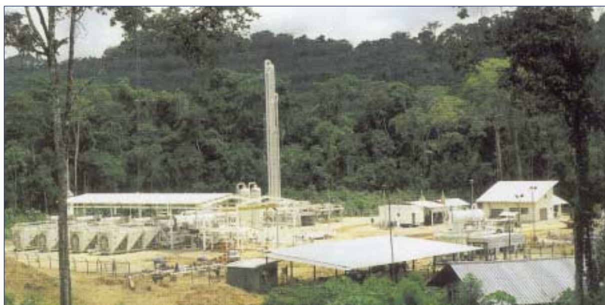
Planta de Separación de Líquidos - Selva Central Liquids Separation Plant – Central Jungle
