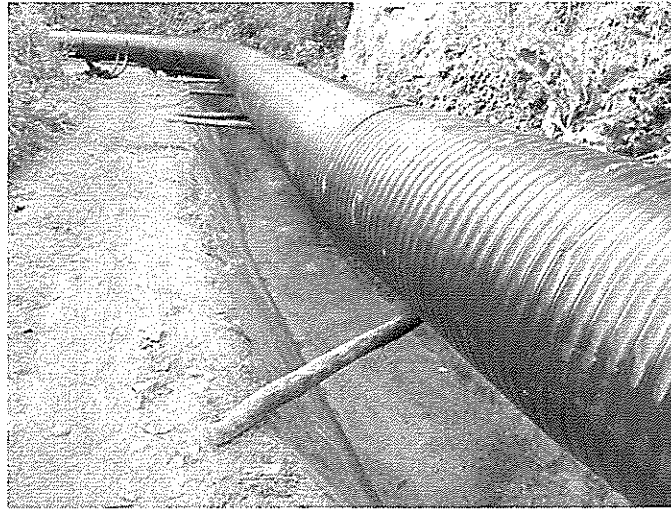
Instalación de Tubería Estructurada PEAD de 900 mm
