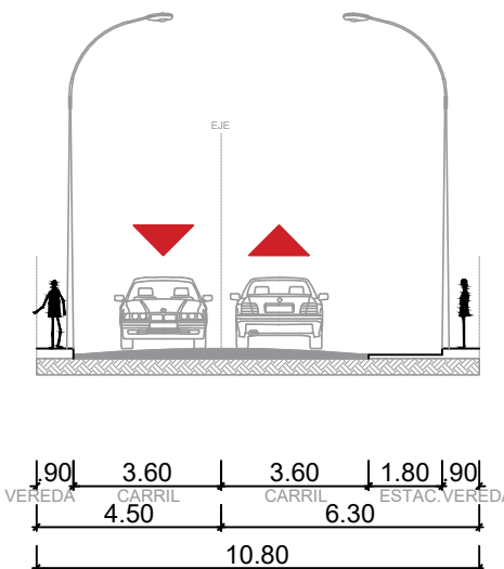
SECCIÓN 5-5 ESC. 1/200
