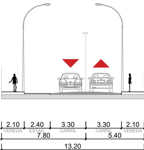
SECCIÓN 2-2 ESC. 1/200
