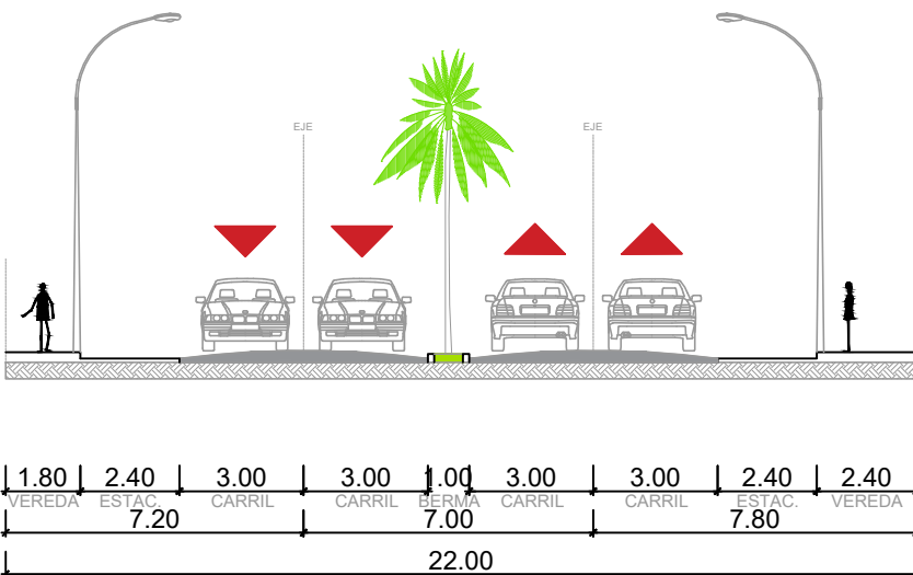
SECCIÓN 4-4 ESC. 1/200
