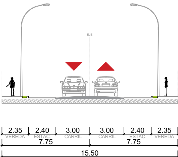
SECCIÓN 3-3 ESC. 1/200
