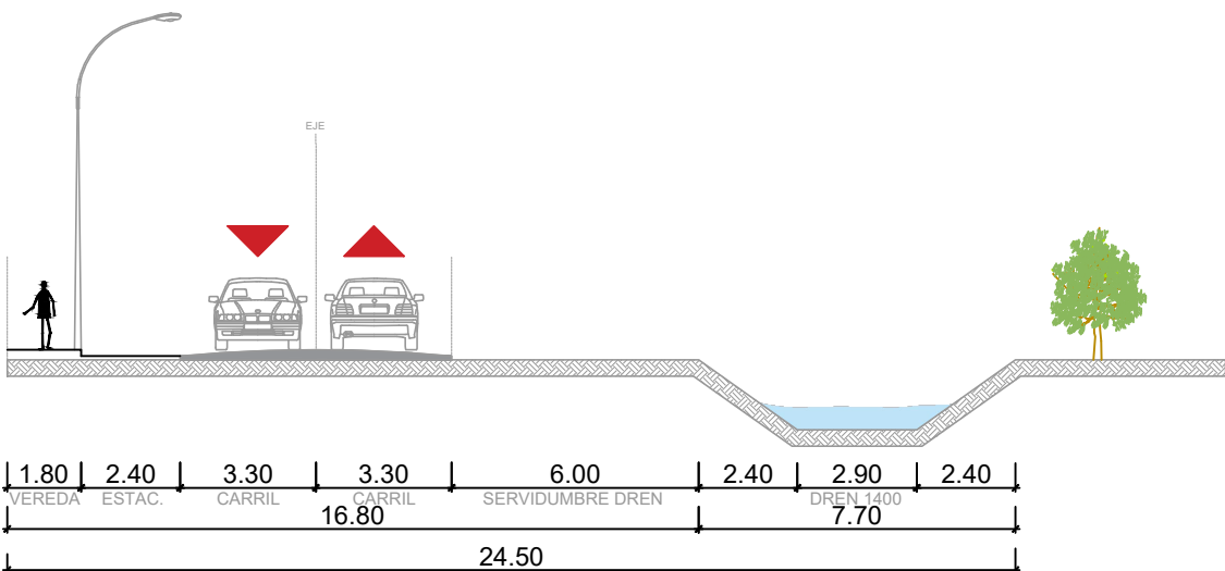
SECCIÓN 1-1 ESC. 1/200
