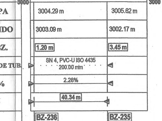
ESC. H: 1/1000 V: 1/200
