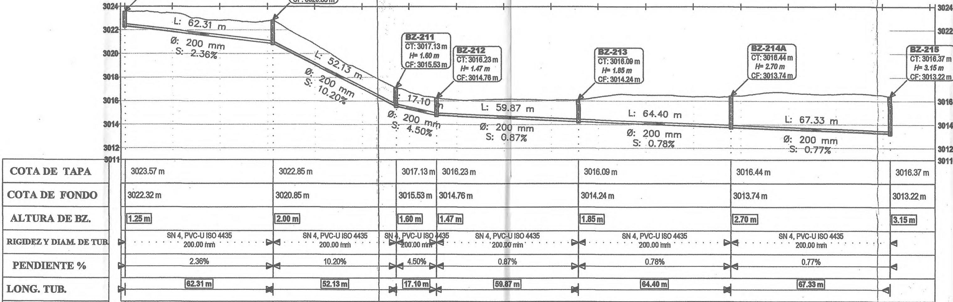
ESC. H: 1/1000 V: 1/200
