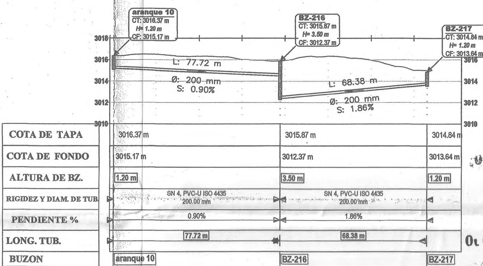
TRAMO: (JR. CHAGLLA entre JR. AMAZONAS Y CURSO DEL RÍO YANAMITO) ESC. H: 1/1000 V: 1/200
