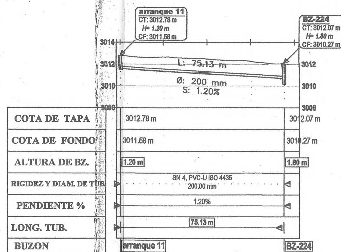
TRAMO: (JR. SANTA ROSA entre JR. AMAZONAS Y JR. SAN AGUSTIN) ESC. H: 1/1000 V: 1/200
