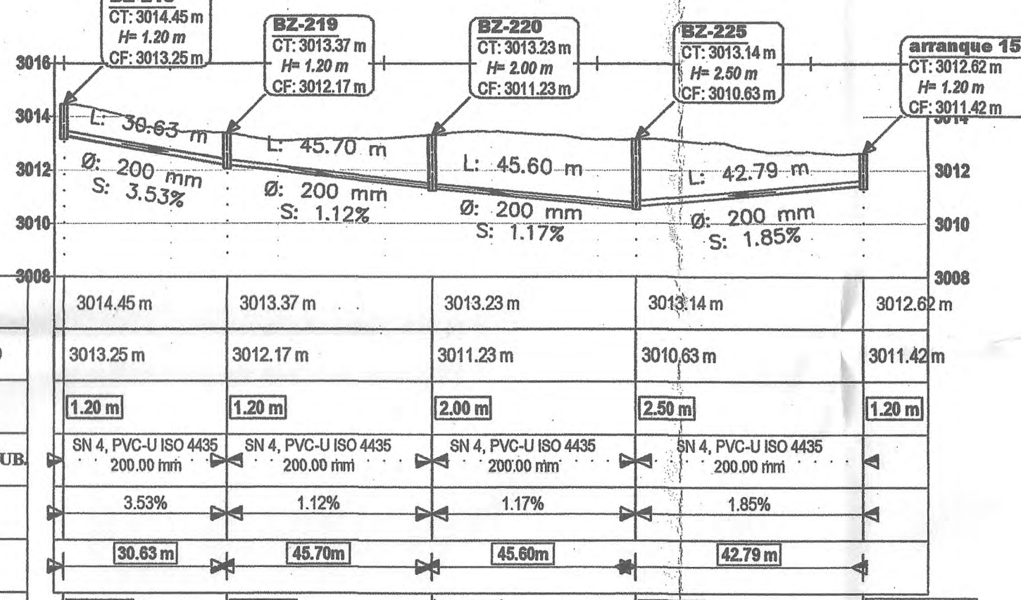
ESC. H: 1/1000 V: 1/200
