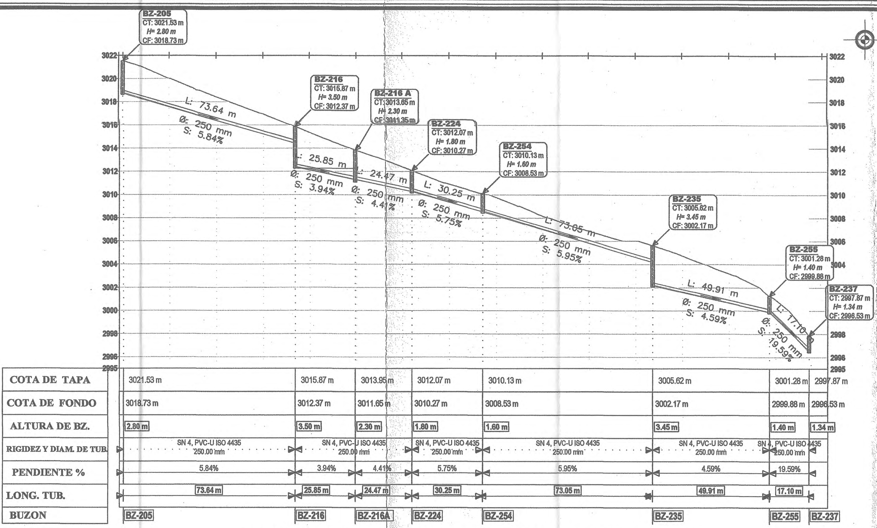
TRAMO: (JR. SAN AGUSTIN entre PROL. MAYRO Y PJE. ESTEBAN BRAVO)
