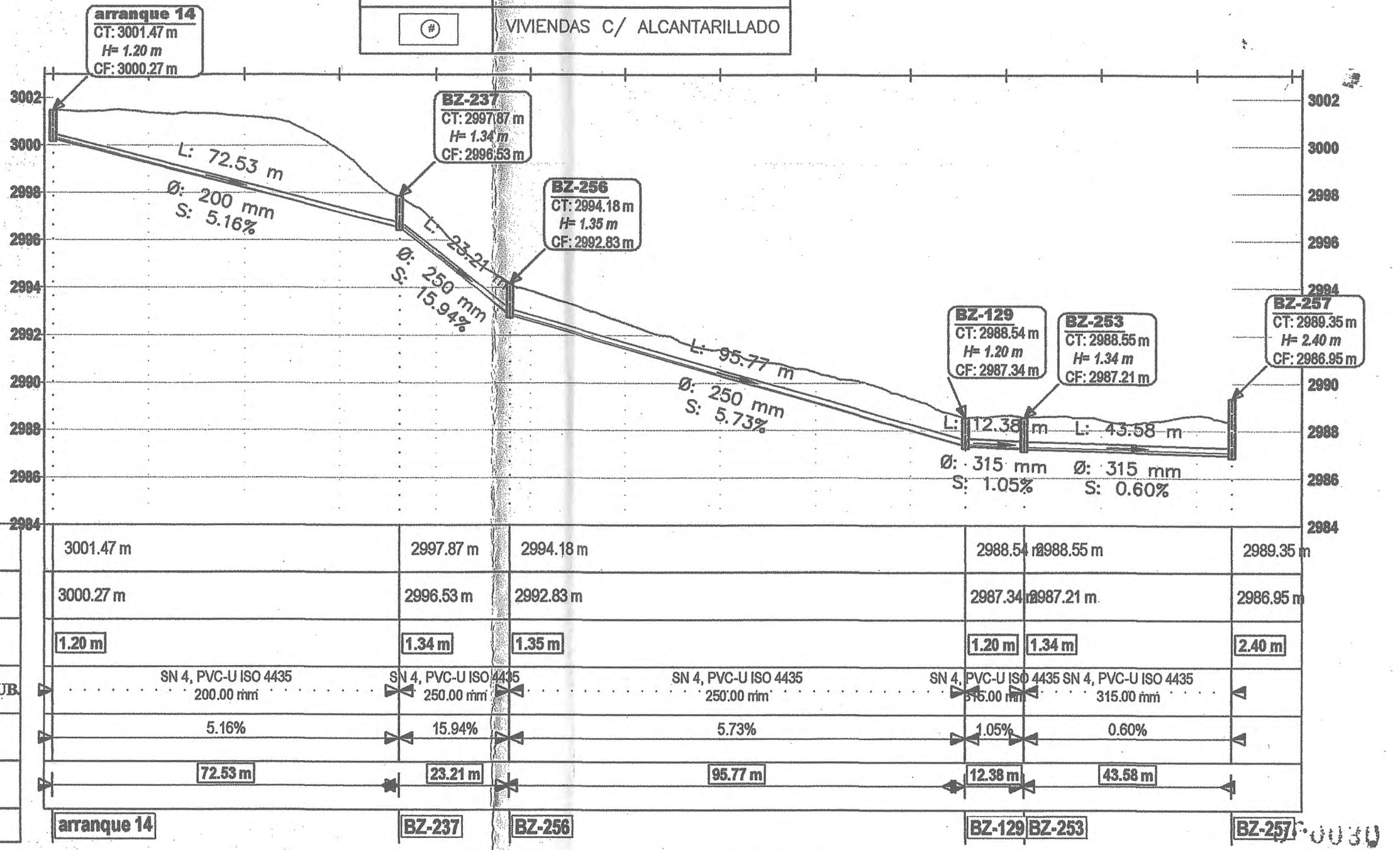
TRAMO: (PJE. ESTEBAN BRAVO Y JR. SAN AGUSTIN)
