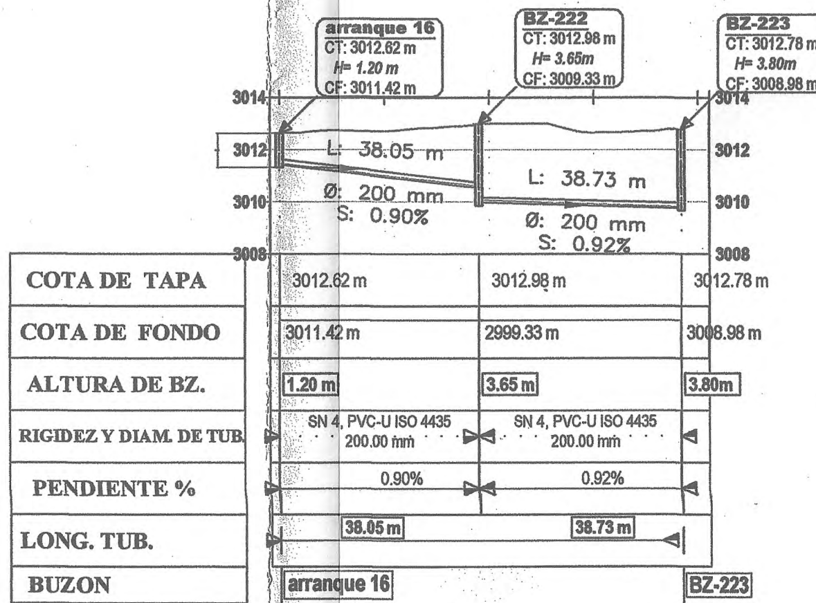
TRAMO: (JR. SANTA ROSA entre JR. SAN JOSÉ Y JR. AMAZONAS) ESC. H: 1/1000 V: 1/200
