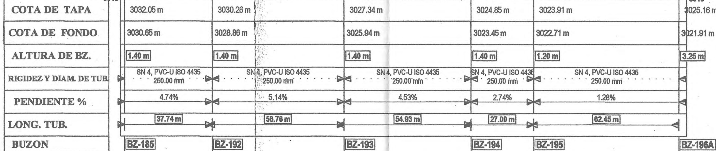
ESC. H: 1/1000 V: 1/200
