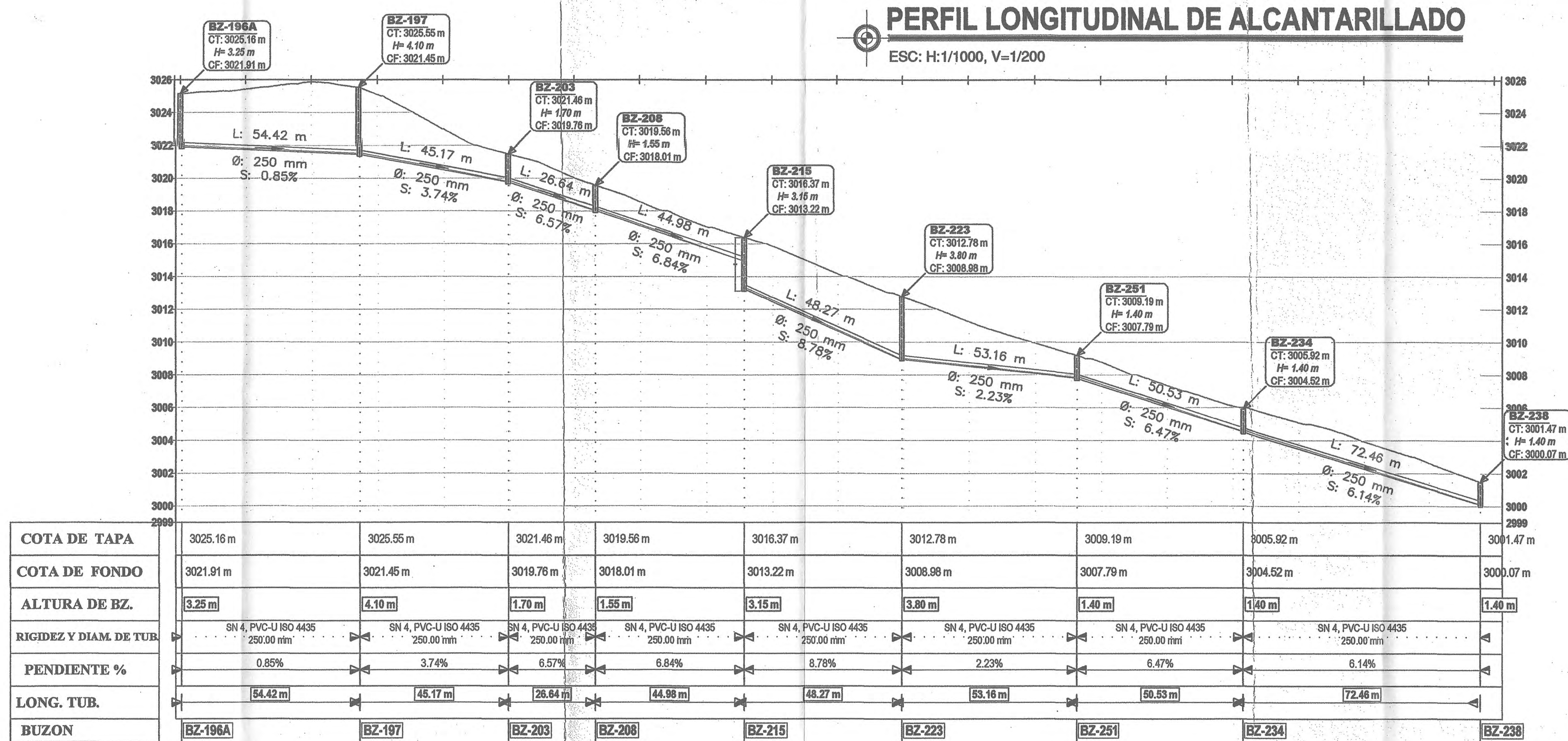
TRAMO: (JR. HUERTAS Y JR. AMAZONAS hasta PJE. ESTEBAN BRAVO) ESC. H: 1/1000 V: 1/200
