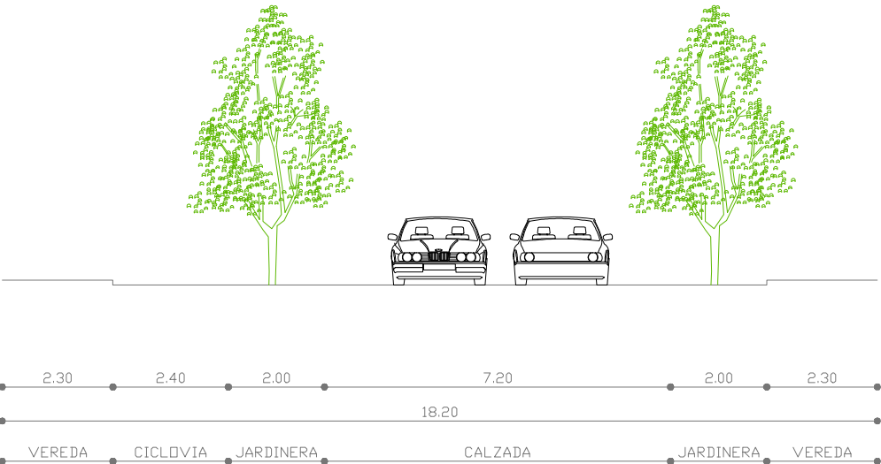
SECCION 2-2 ESC:1/200
