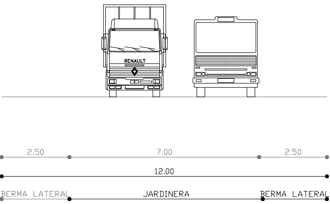
SECCION 1'-1' ESC:1/200
