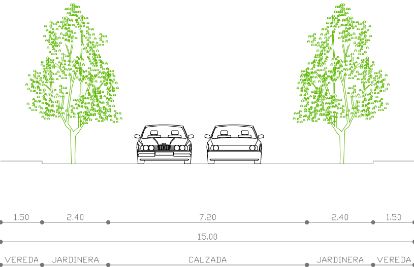
SECCION 3-3 ESC:1/200
