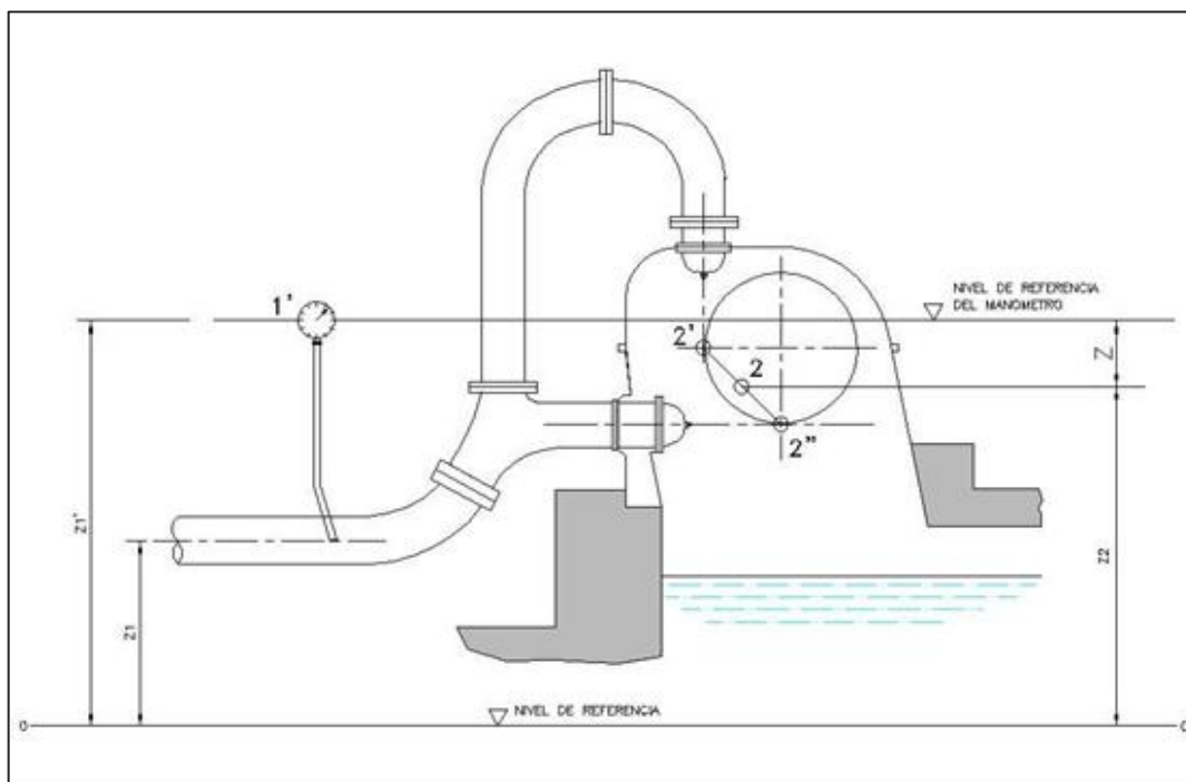
Figura N° 3. Turbina Pelton de eje horizontal (Referencia IEC 60041)
