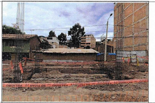
Colocado de acero para columnas en caseta de Sub estación N° 02.
