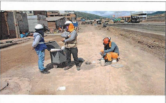
Pruebas de Densidad de campo en base granular en el Km. 4+100 carril auxiliar izquierda.
