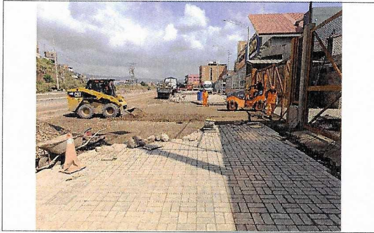
Mejoramiento de base para veredas en la progresiva 6+600.
