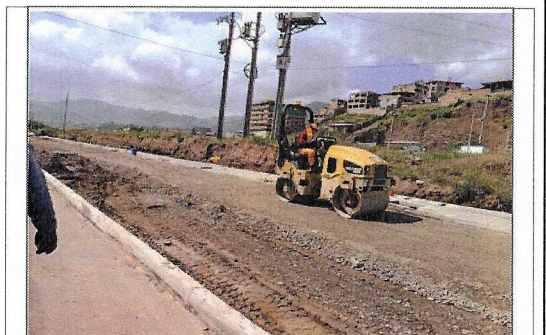
Mejoramiento de base para ciclovía en el Sector Versalles.
